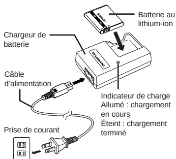
Chargeur de batterie LI-50C
