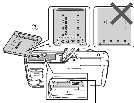
Akkuverriegelung
