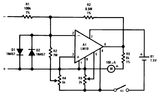
Meter Amplifier
