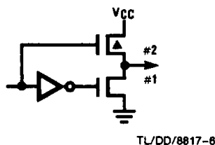
a. Standard Output
