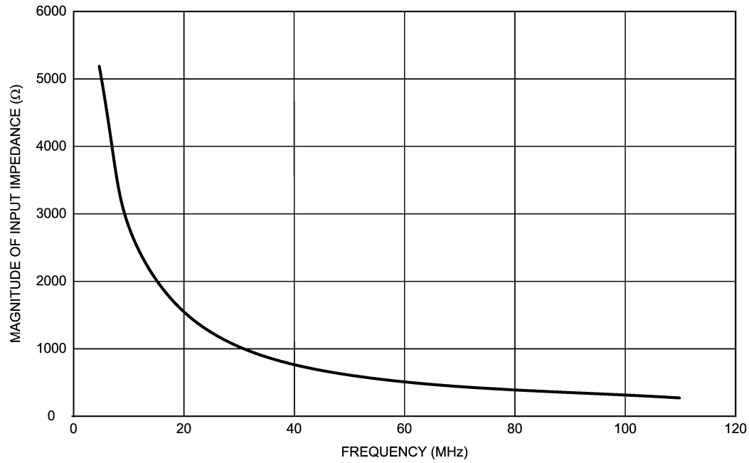
OSCin Input Impedance ( V_{CC}=2.5\text{ V} , T_A=25\text{ }^{\circ}\text{C} ) (Note 5)
