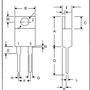
TO-220A
