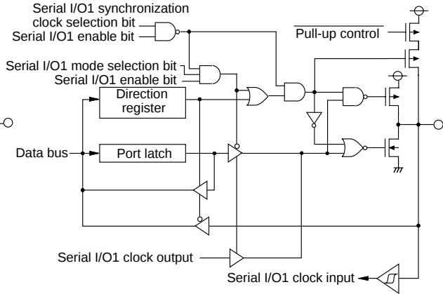
(7) Port P46
