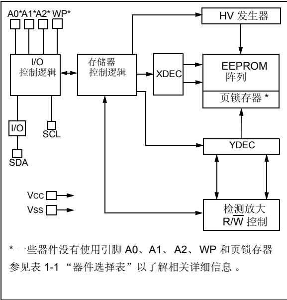
原理框图
