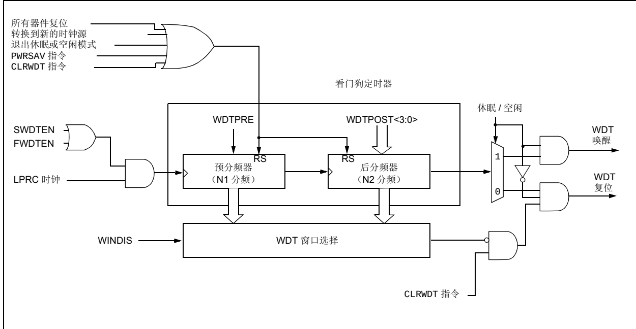
图 21-2: WDT 框图
