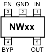
MIC5256-x.xBD5 (TSOT-23-5)
