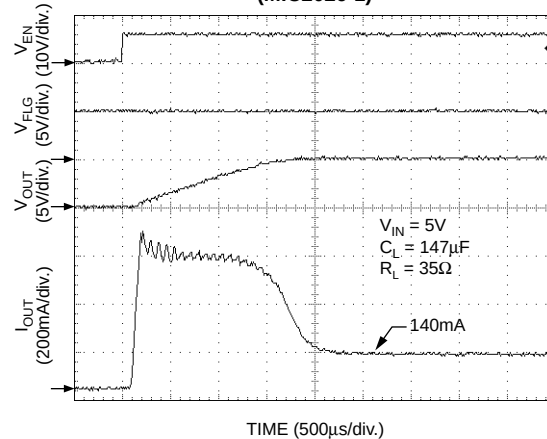
Turn-On (MIC2026-1)
