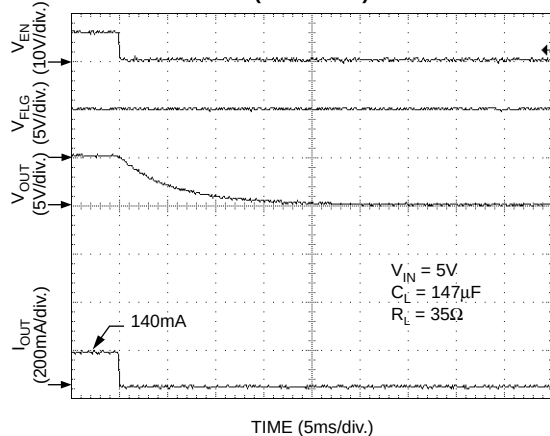
Turnoff (MIC2026-1)
