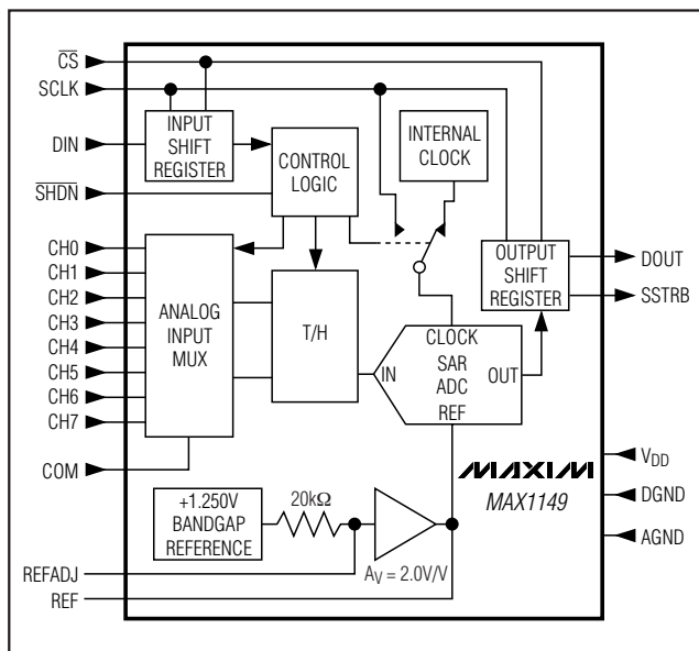
图 5. 原理图
