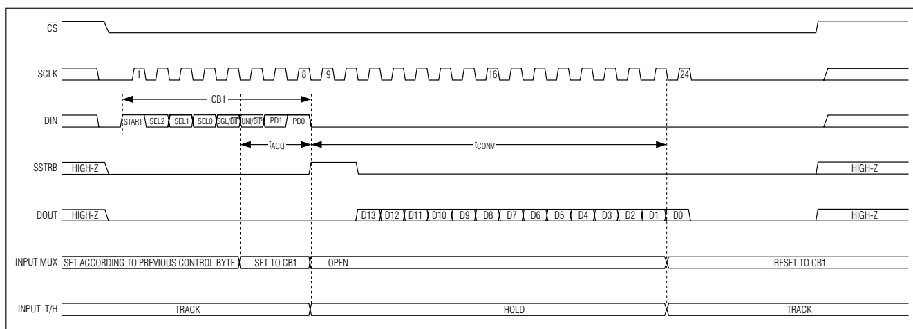
图 8. 外部时钟模式 — 24 时钟/转换时序
