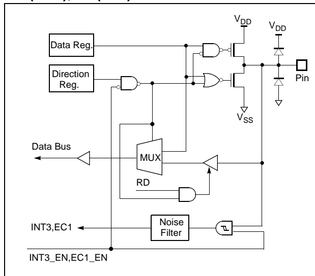
R50(INT3), R51(EC1)
