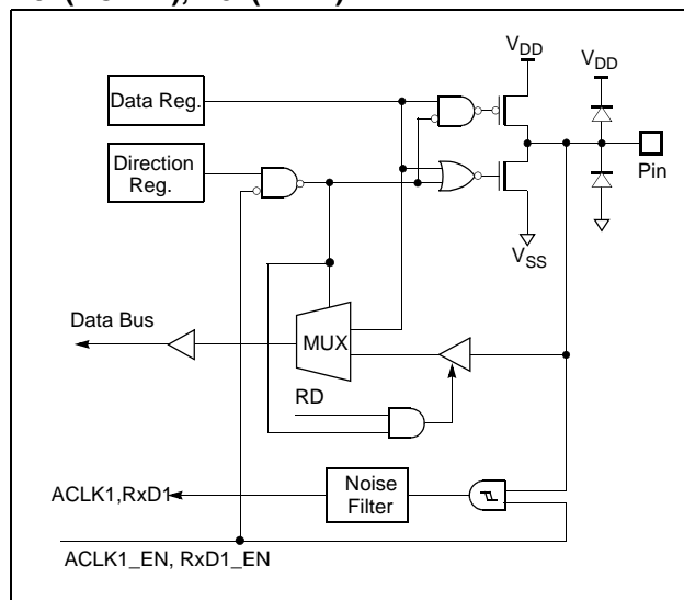
R31(ACLK1), R32(RxD1)
