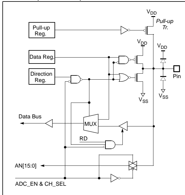
R70~R77(AN8~AN15)
