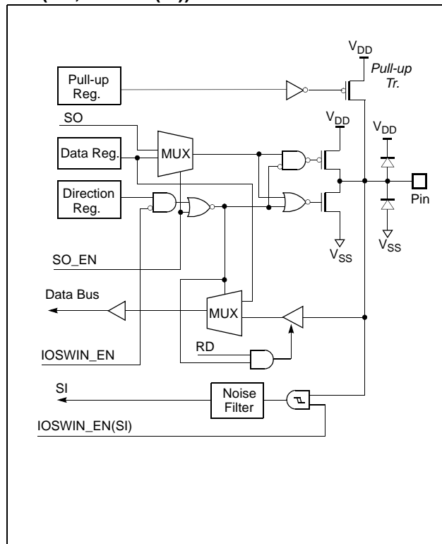
R44(SO, IOSWIN(SI))
