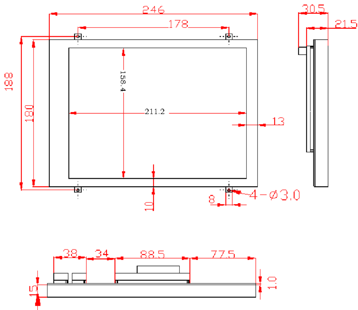
LR104AR/B系列液晶显示器金属板安装尺寸图
