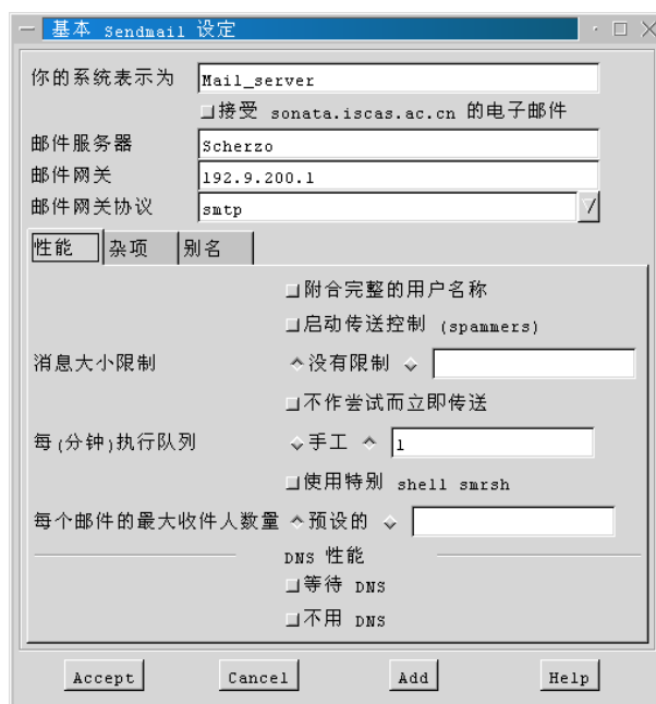
图 4-14. 配置 sendmail
