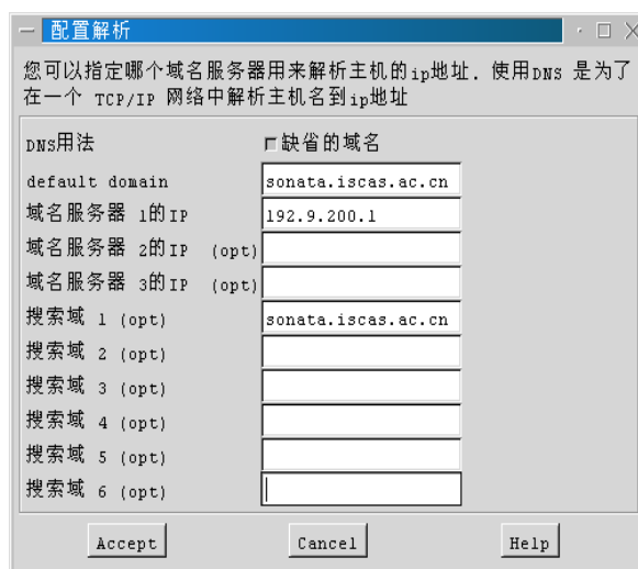
图 4-7. 配置解析
