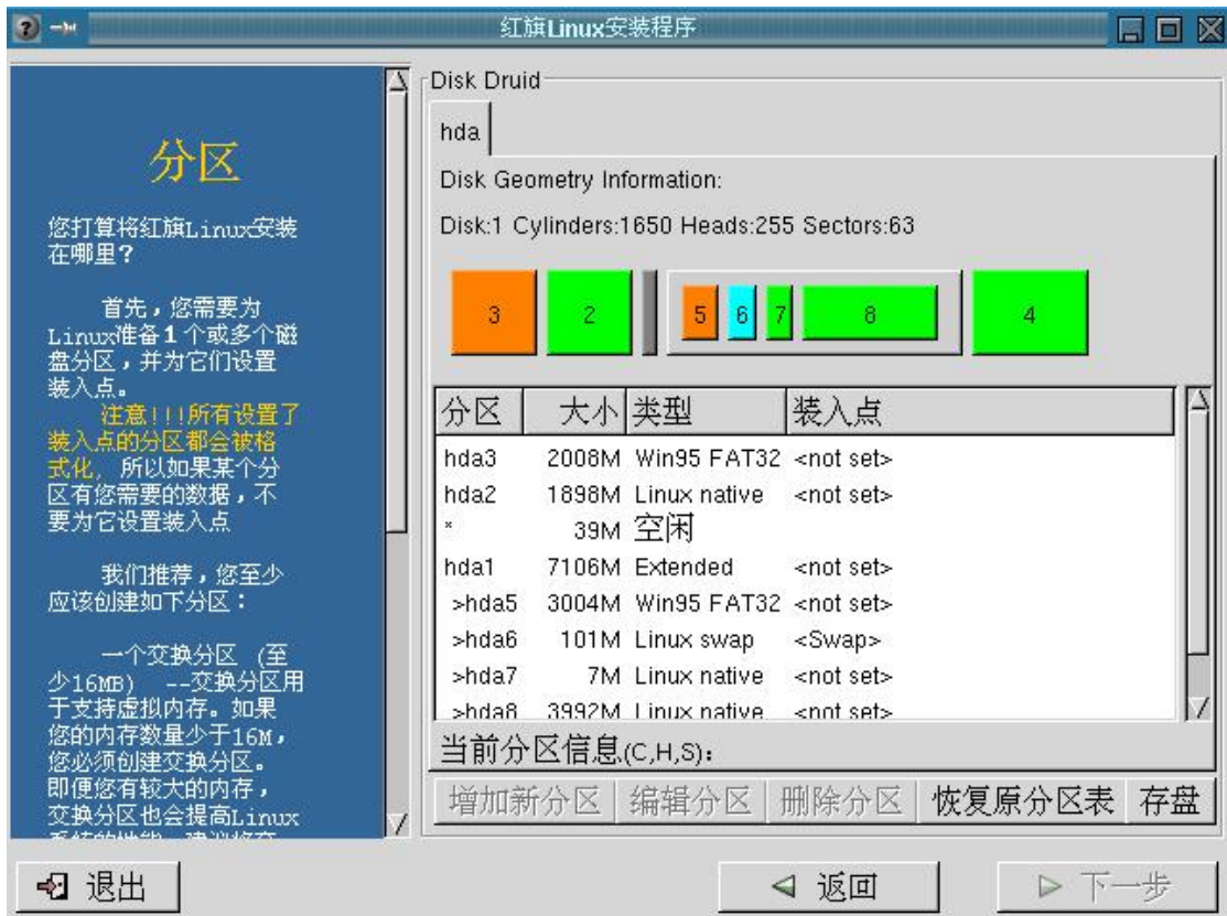
图 1-6. 手工分区
