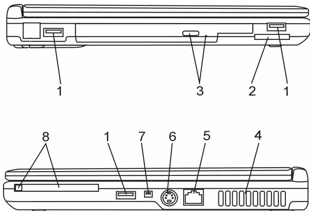
侧视图
