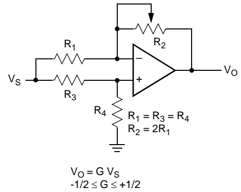
Attenuator
