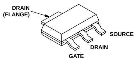
SOT-223
