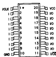
SOIC
