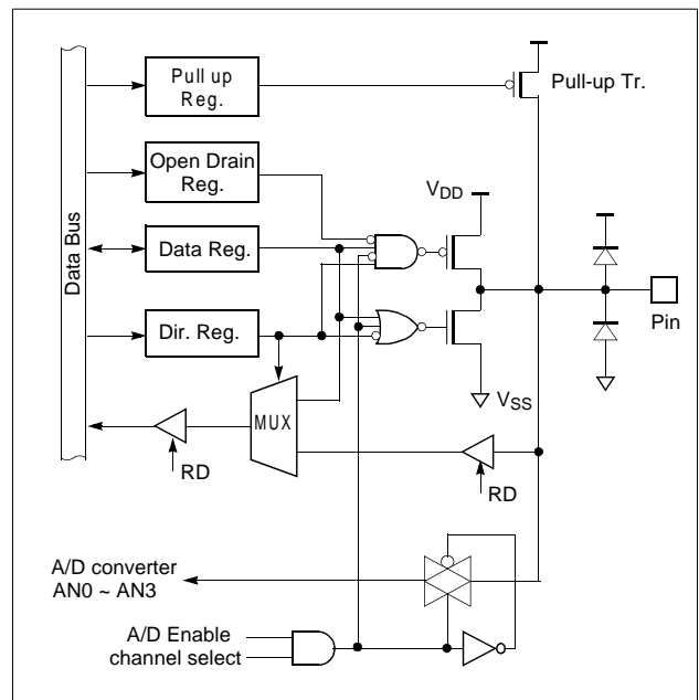
R20~R23/AN0~AN3
