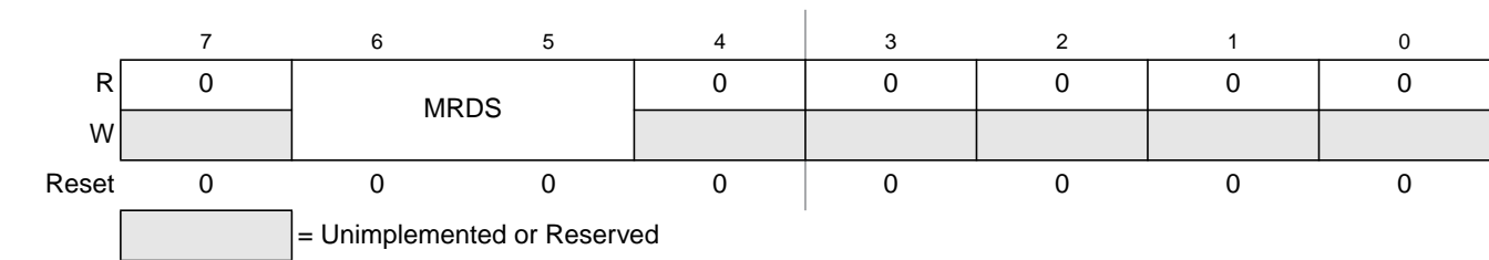
Figure 29-6. Flash Test Mode Register (FTSTMOD)
