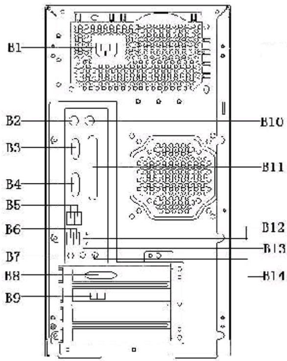
主机后面板
