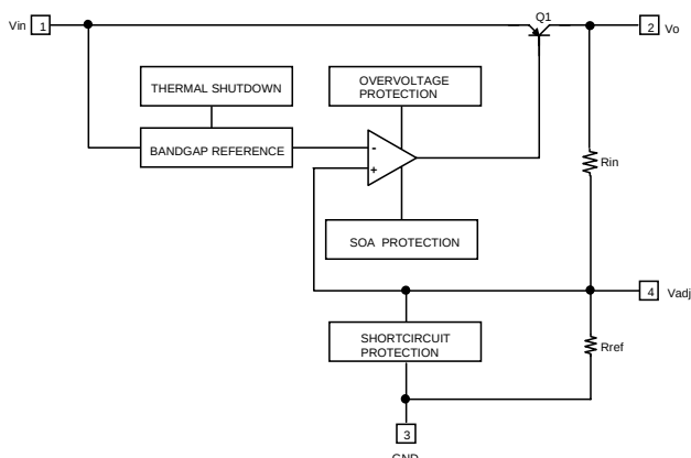
(KA278RA05C)
