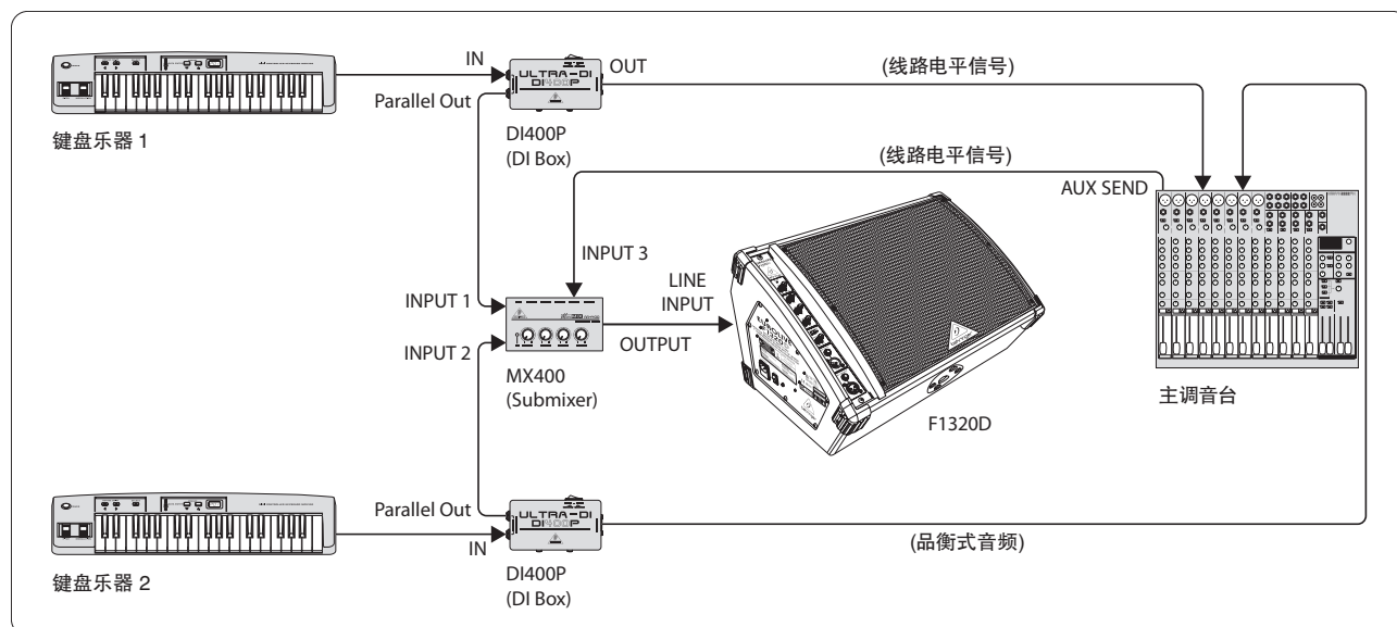
图 3.1 F1320D 与 2 个键盘乐器同时使用
