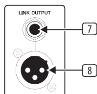
图 2.4 LINK OUTPUT
