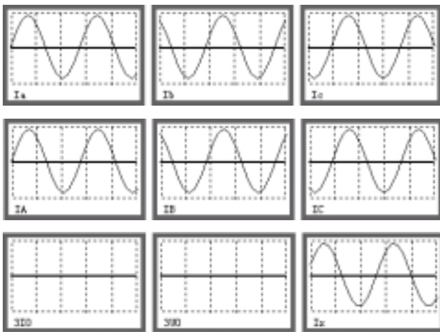
图 3.3.5 实时波形图显示画面
