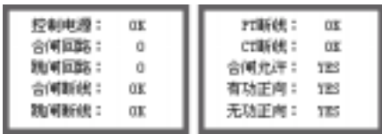
图 3.3.8 调试信息显示画面
