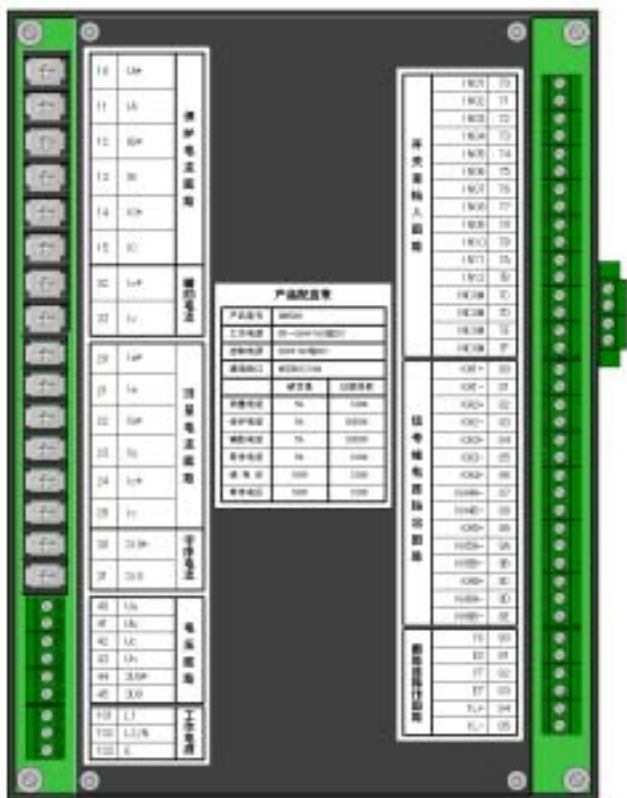
图 2.2 DMR261 后面板接线端子图
