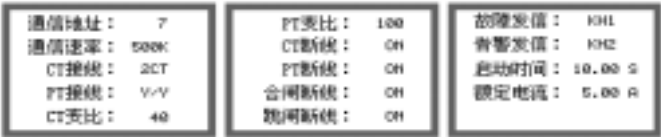
图 3.3.10b 线路参数显示画面
