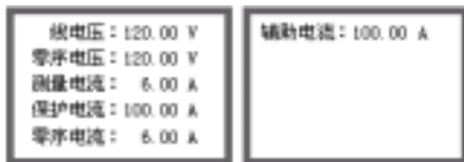
图 3.3.10e 二次测量量程显示画面
