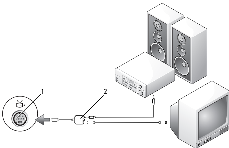
1 S-video 电视输出连接器
