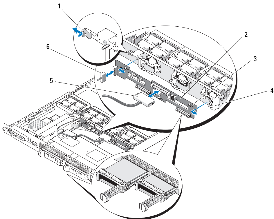
图 3-23. 卸下和安装 2.5 英寸硬盘驱动器背板
