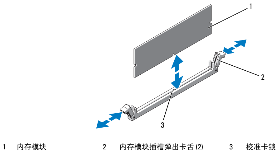
图 3-13. 安装和卸下内存模块
