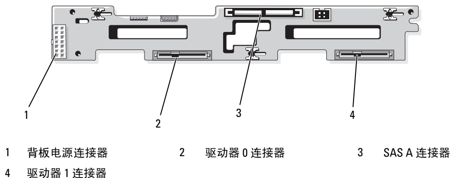
图 6-3. SAS 3.5 英寸驱动器背板组件 — 选件 1
