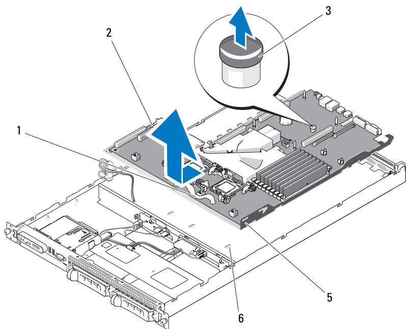
图 3-26. 卸下系统板
