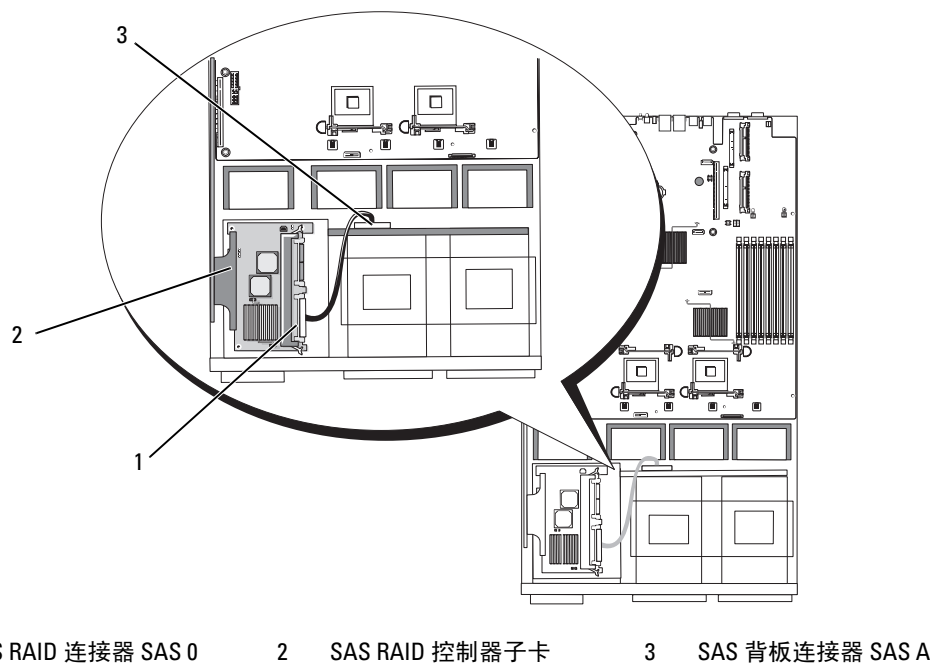
图 3-10. CSAS RAID 控制器子卡的电缆路径
