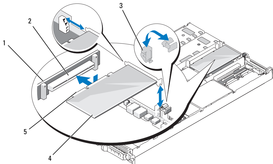
图 3-12. 安装扩充卡
