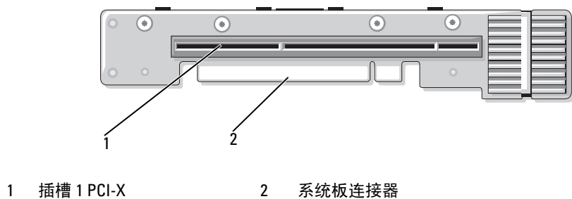
图 6-7. 可选 PCI-X 扩充卡中央提升板组件
