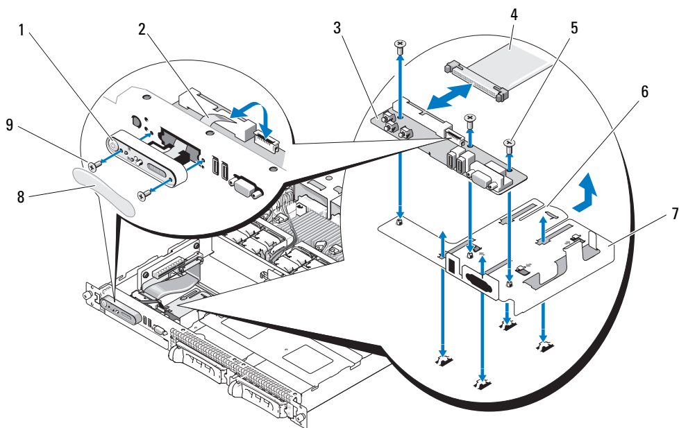
图 3-25. 卸下和安装控制面板
