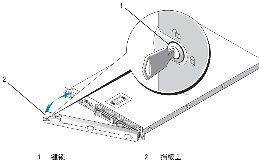
图 3-2. 卸下挡板
