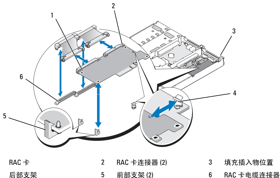
图 3-16. 安装 RAC 卡
