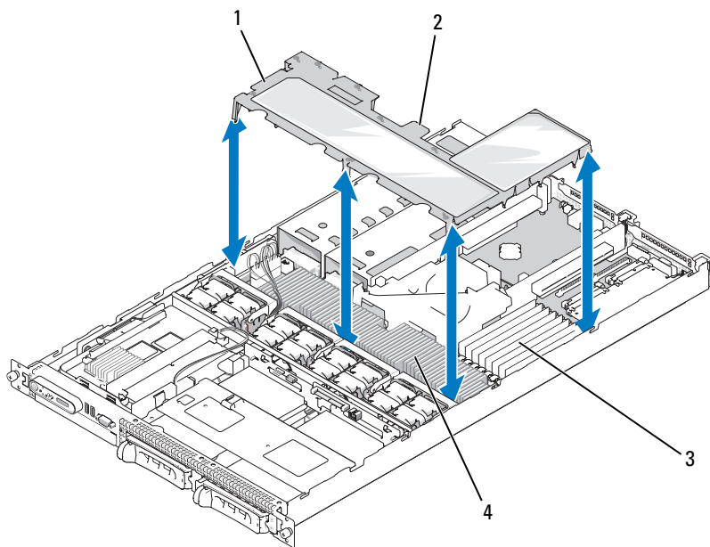
图 3-6. 内存冷却导流罩
