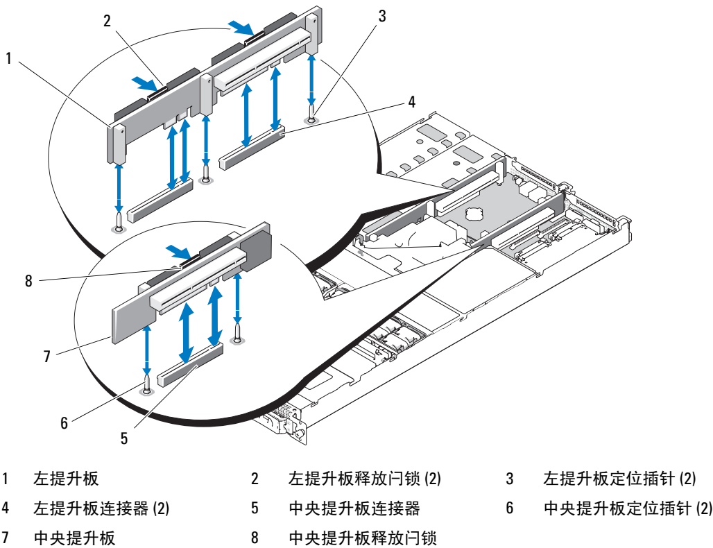
图 3-22. 卸下扩充卡提升板
