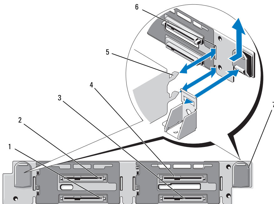
图 6-4. SAS 2.5 英寸驱动器背板组件 — 选件 2（正面）
