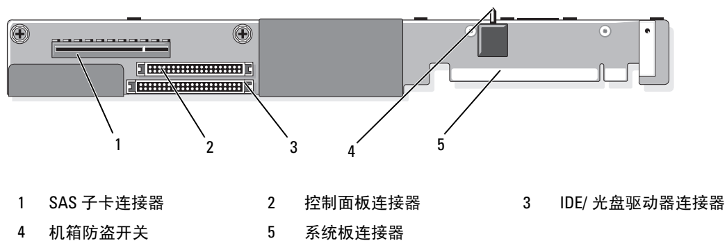
图 6-8. 侧板组件
