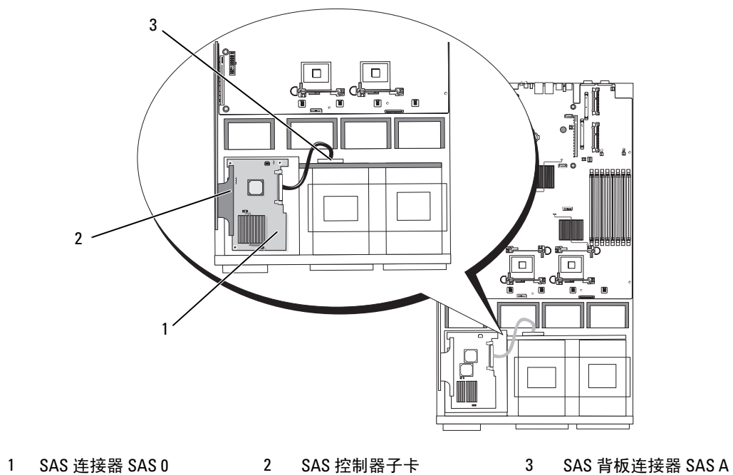
图 3-9. SAS 控制器子卡的电缆路径
