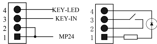
图3-2-3 4PIN接口定义及外部接法
