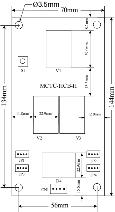
图3-3-10 安装尺寸
