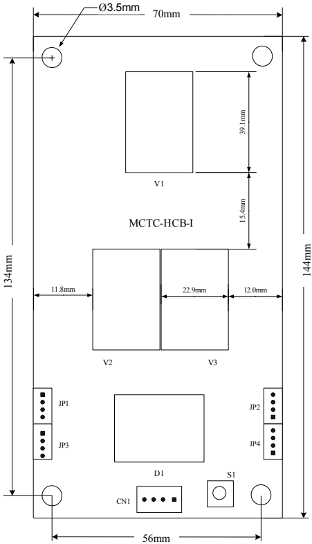
图 3-3-12 MCTC-HCB-I安装尺寸
