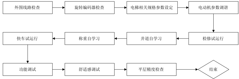
图7-1 调试流程
