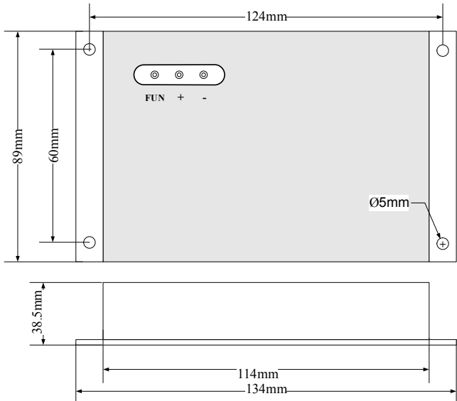
图 3-6-1 MCTC-CHM-B 尺寸图
