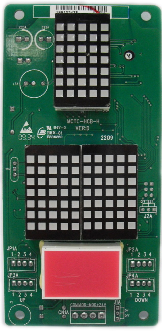
图3-3-9 MCTC-HCB-H实物图
