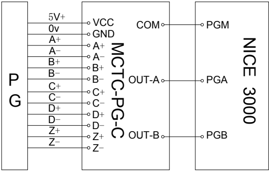
图4-10 MCTC-PG-C接线图（ERN1387型编码器）
