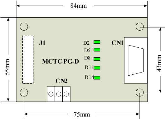
图4-8 MCTC-PG-D外观及尺寸
