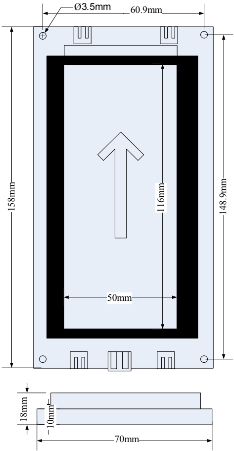
图3-3-6 MCTC-HCB-D1尺寸图
