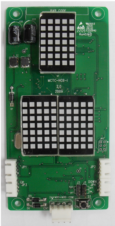
图 3-3-11 MCTC-HCB-I实物图
