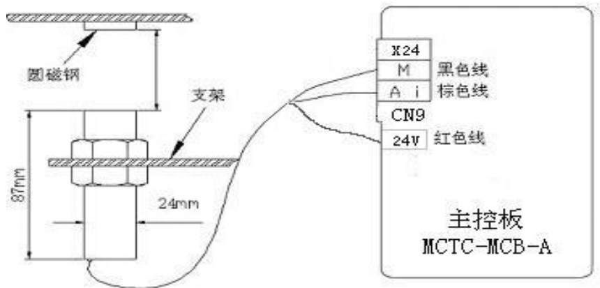
图3-7-2称重传感器安装示意图(传感器接主控板)
