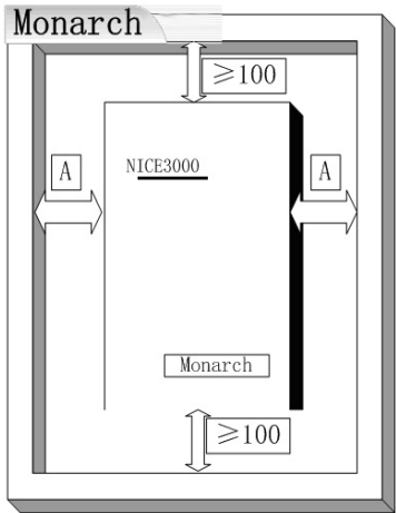
图4-2 控制器的安装尺寸要求
