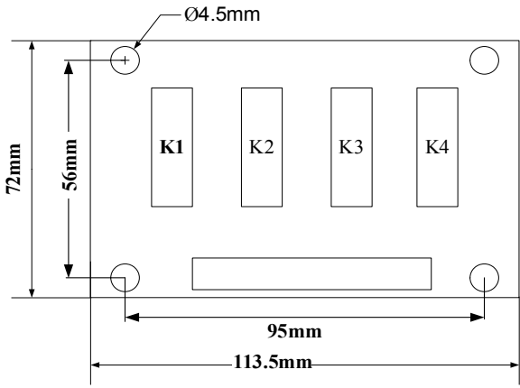
图3-5-2外观尺寸图
