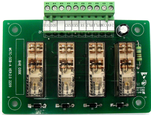
图3-5-1 实物图
