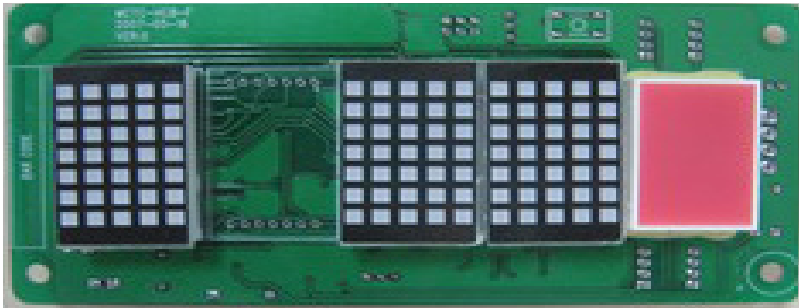
图 3-3-7 MCTC-HCB-F实物图
