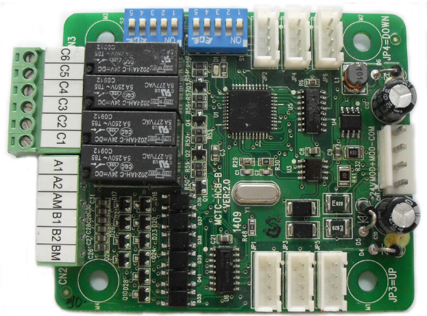
图 3-3-1 MCTC-HCB-B实物图
