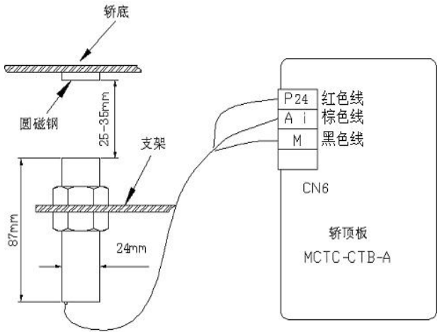
图3-7-1称重传感器安装示意图(传感器接轿顶板)
