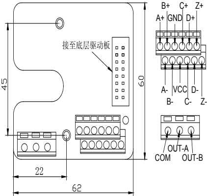
图4-9 MCTC-PG-C（ERN1387型编码器）
