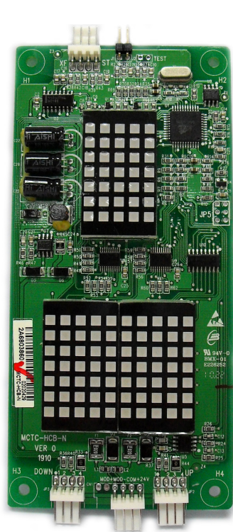
图3-3-13 MCTC-HCB-N实物图
