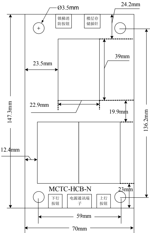
图3-3-14 MCTC-HCB-N安装尺寸
