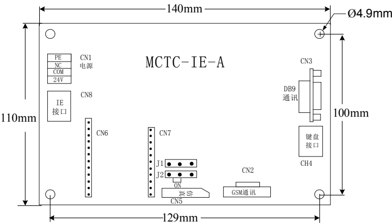
图3-8-1 MCTC-IE-A安装尺寸图
