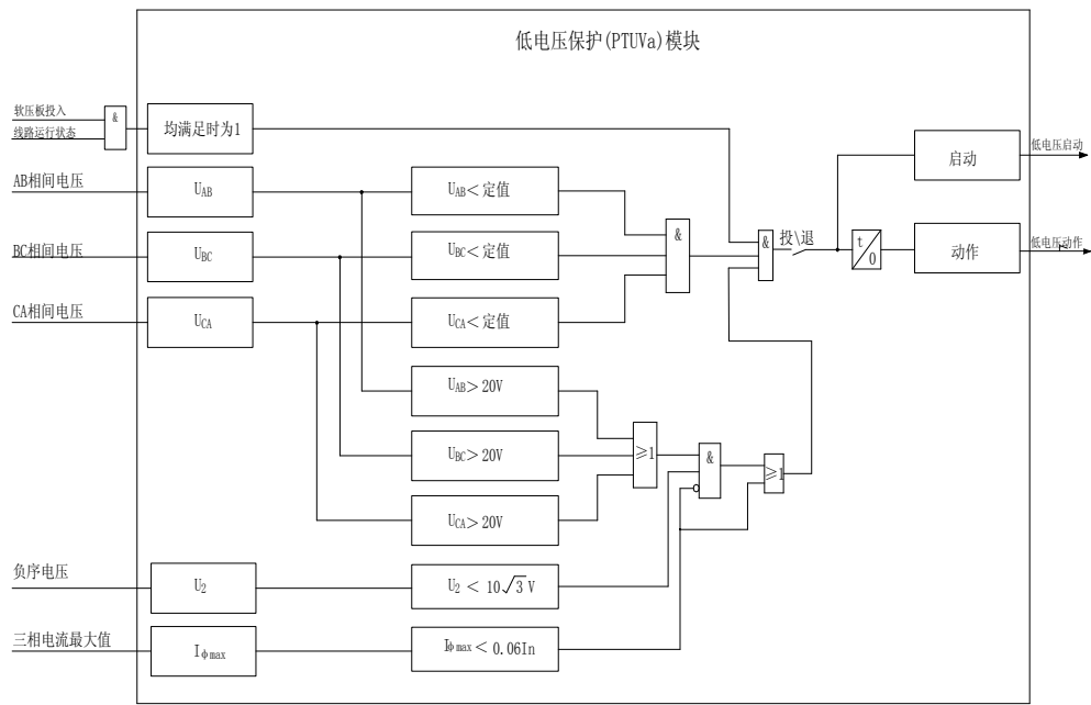
图4-16 低电压保护原理框图
