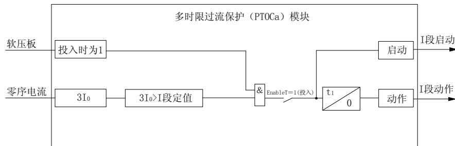
图4-9 高压侧I段零序过流保护原理框图（II段同I段）
