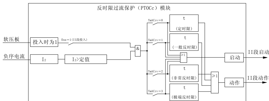
图4-7 II段负序过流保护原理框图
