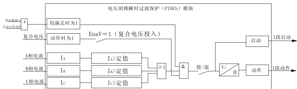
图4-3 I段复合电压过流保护原理框图 (II段同I段)
