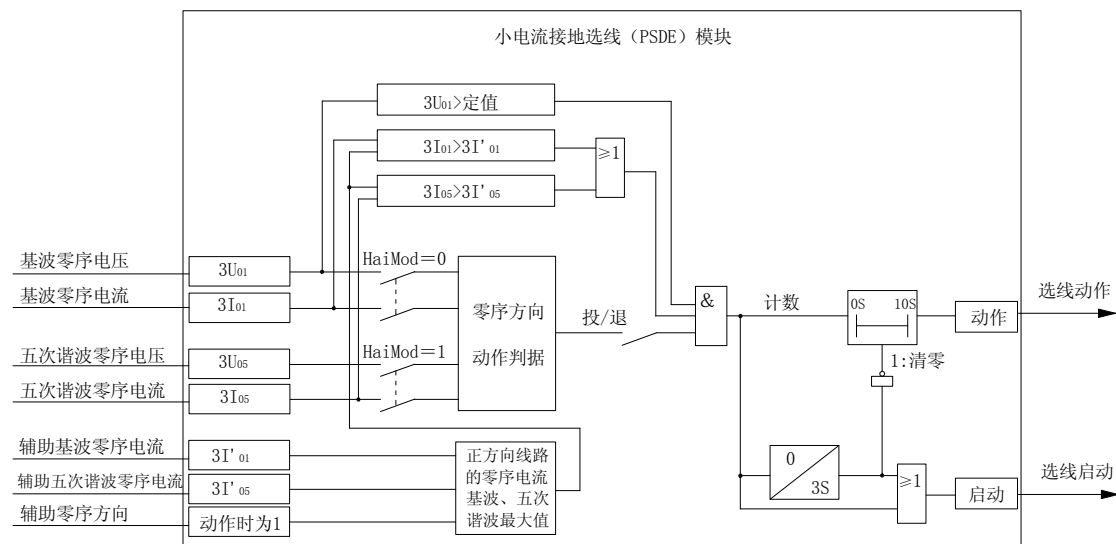
图4-15 小电流接地选线原理框图
