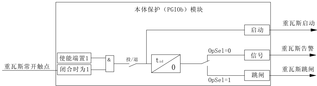
图4-17 重瓦斯本体保护原理框图（其它本体保护原理与重瓦斯相同）
