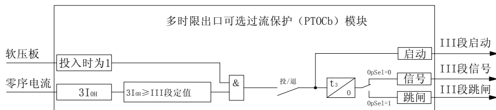
图4-10 高压侧III段零序过流保护原理框图
