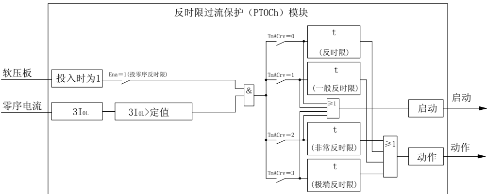
图4-13 低压侧零序反时限过流保护原理框图
