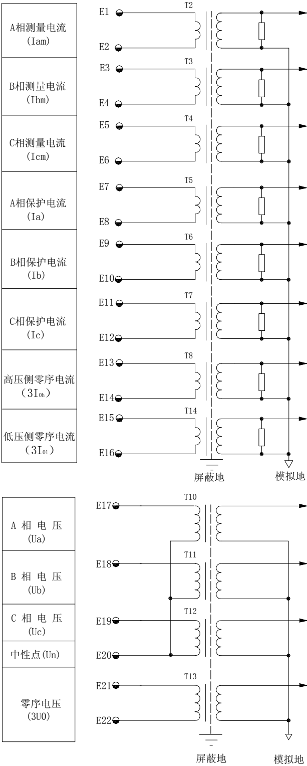
附图1 DSI 5115交流回路原理图
