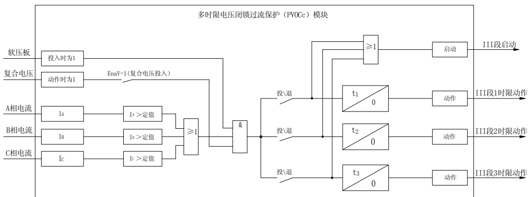
图4-4 III段复合电压过流保护原理框图
