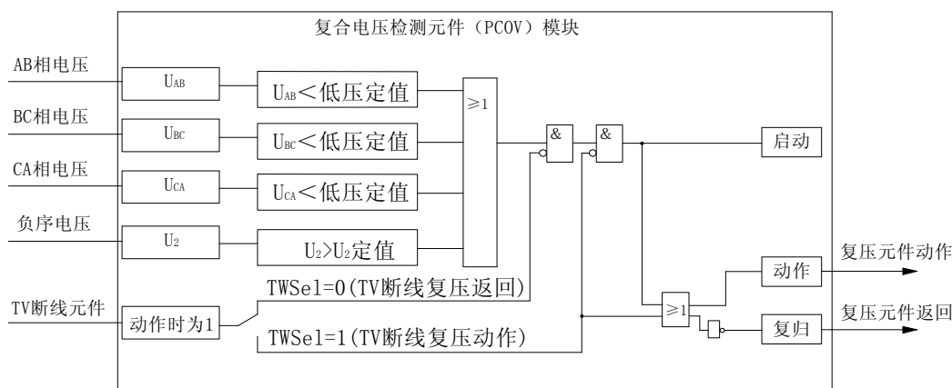
图4-2 复合电压元件原理框图
