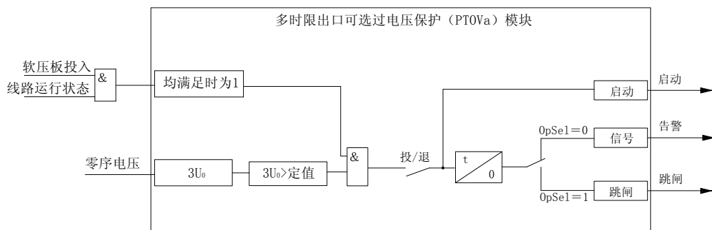
图4-14 零序过压保护原理框图
