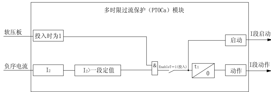
图4-6 I段定时限负序过流保护原理框图
