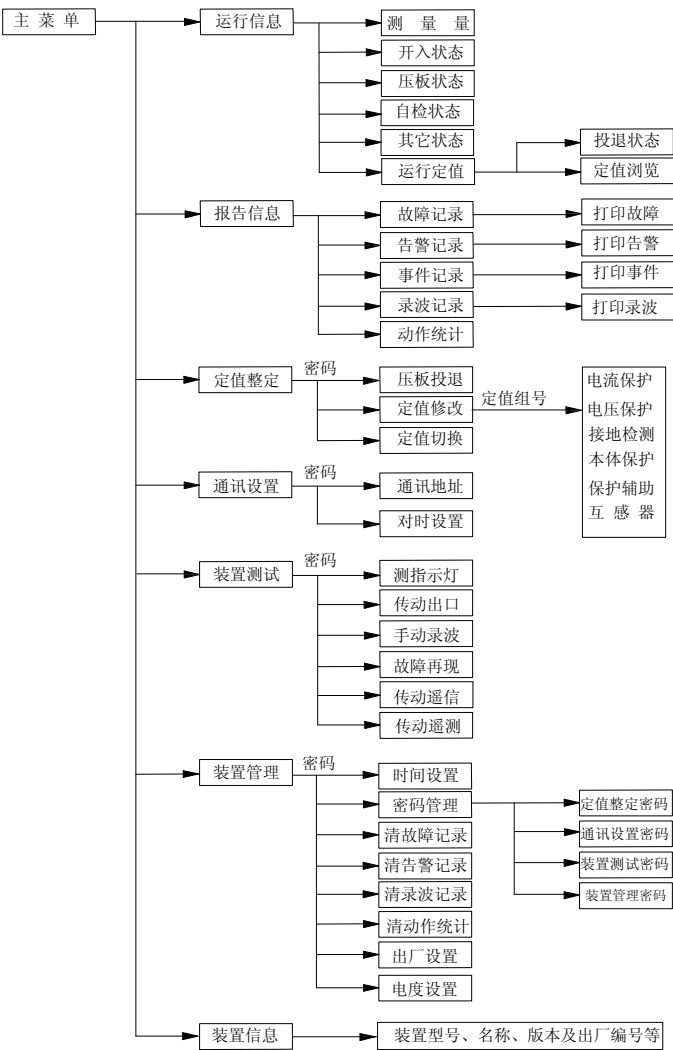
图5-4 液晶界面拓补图
