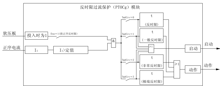
图4-5 正序反时限过流保护原理框图
