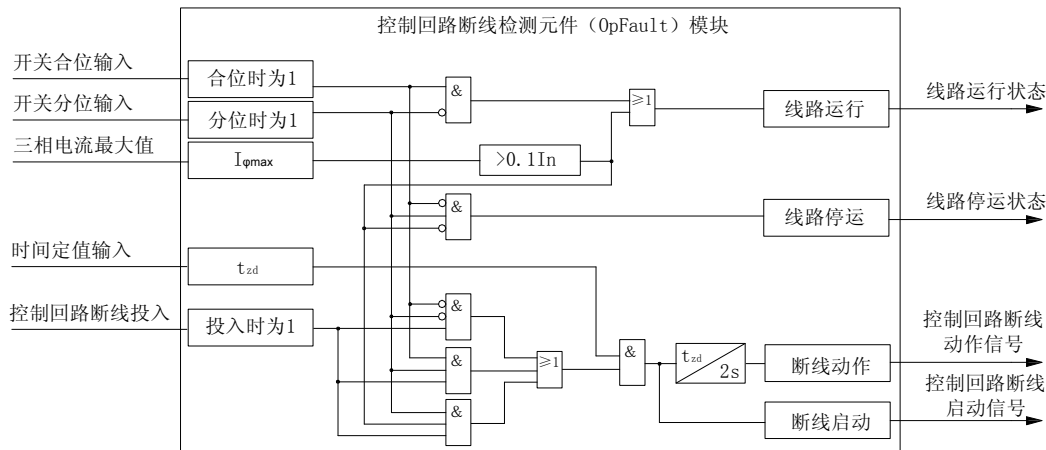
4-19 控制回路断线检测及线路状态监视功能原理框图
