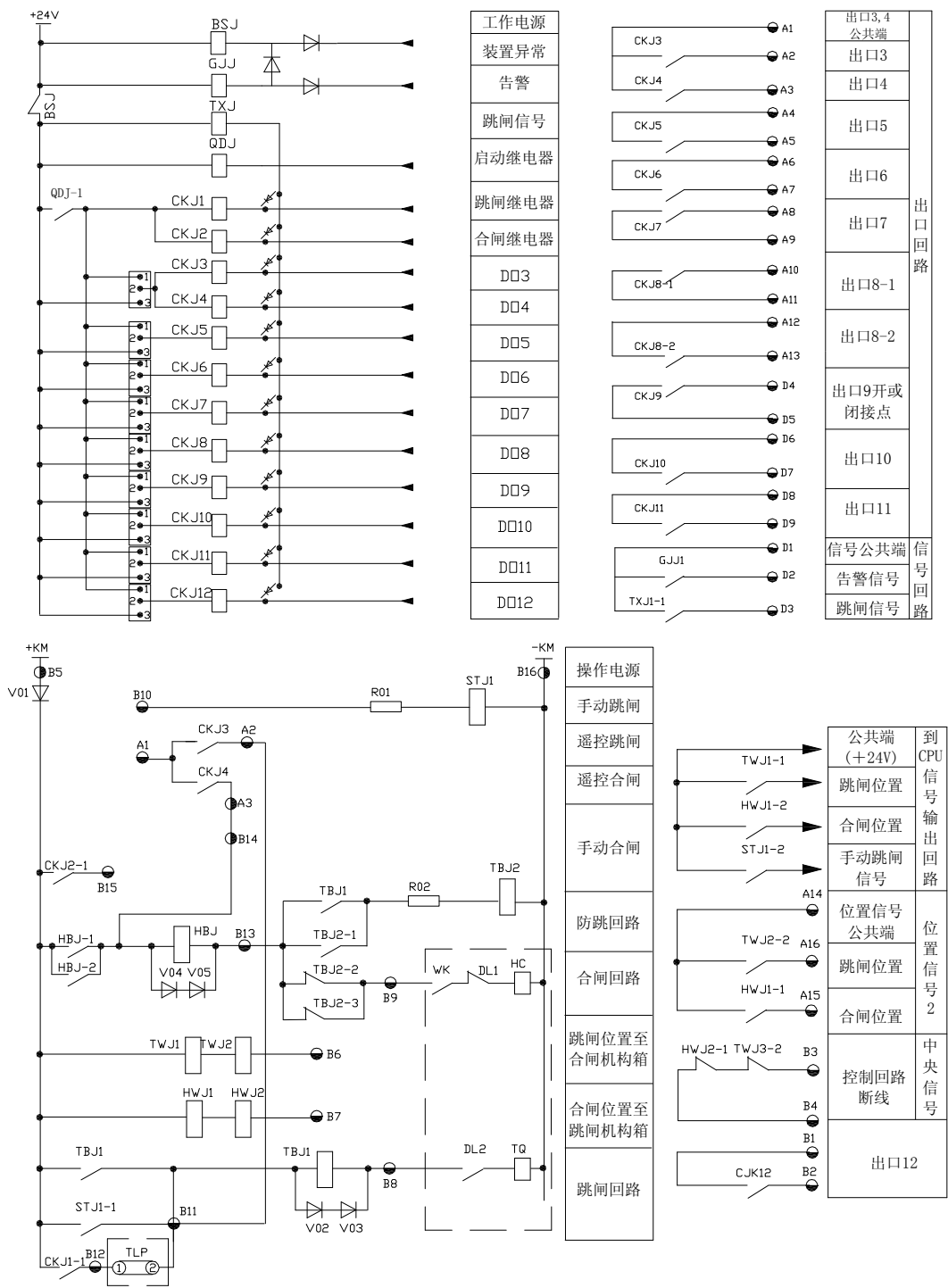
附图2 DSI 5115出口及操作回路端子图
