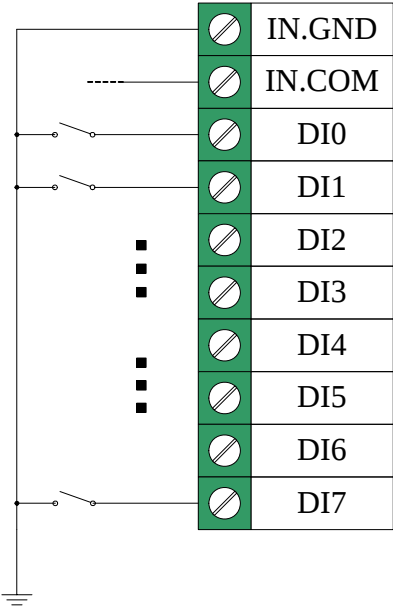
图2.4-1 干接点
