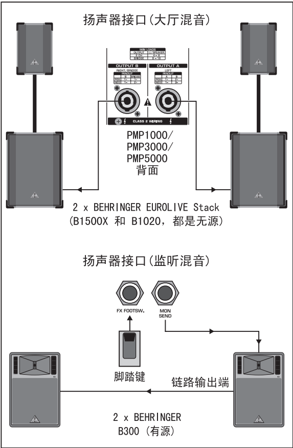
图 5.1: EUROPOWER 调音台作为立体声放大器
