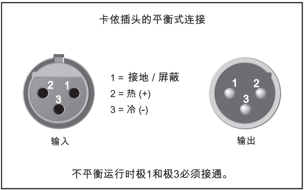
图 4. 3: XLR 连接
