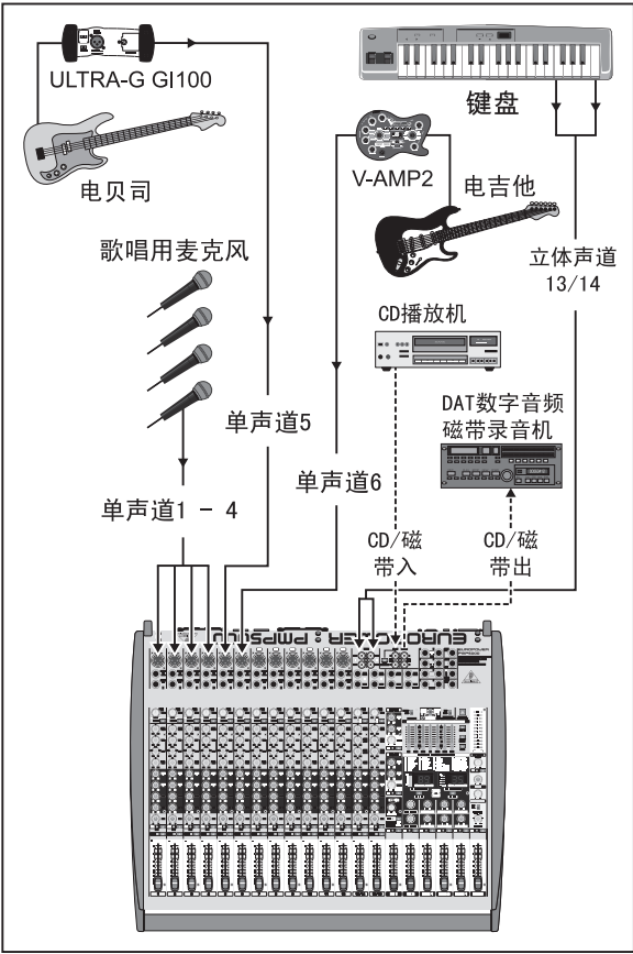
图 5. 4: 标准设置 (举例)
