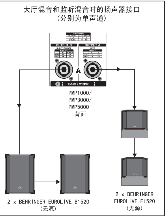
图 5. 3: EUROPOWER 调音台作为单声双通道放大器 (举例)
