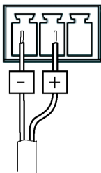
Gleichstromeingang
