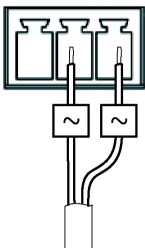
Wechselstromeingang
