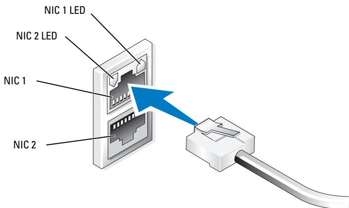
图 1-1. NIC 连接器
