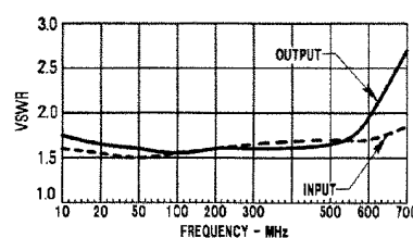
VSWR
