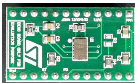
STEVAL-MKI074V1
