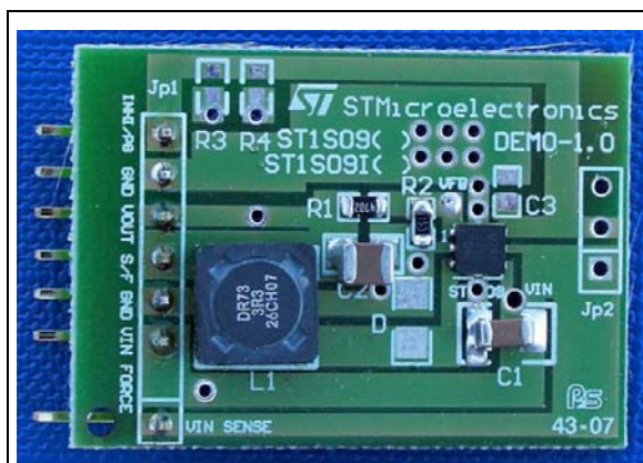
STEVAL-ISA046V2
