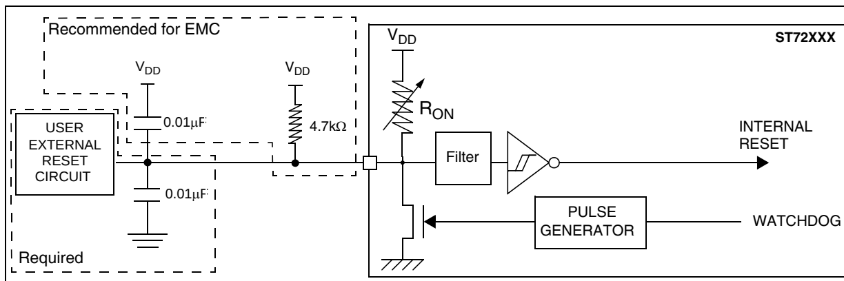
Figure 74. \overline{\text{RESET}} pin protection 1)2)3)4)
