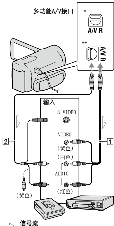
信号流
