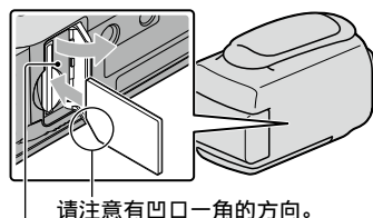
存取指示灯
