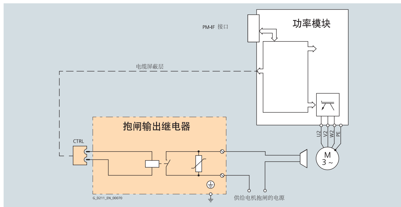
抱闸输出继电器的连接
