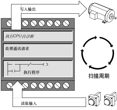
图8-5 S7-200扫描周期
