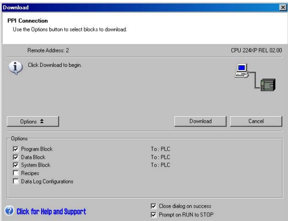
图4-13 下载程序到S7-200 CPU
