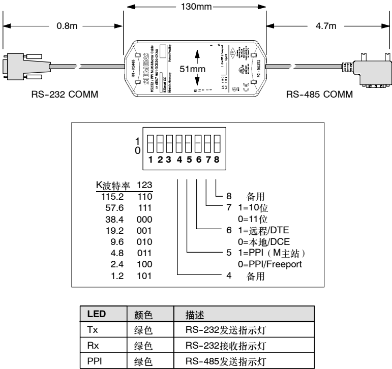
图A-41 S7-200 RS-232/PPI多主站电缆的尺寸、标签和LED
