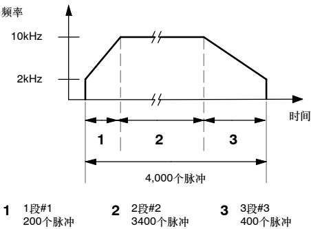
图6-31 频率/时间图
