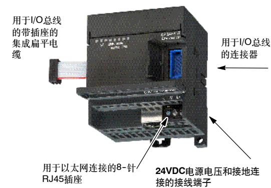
图A-38 连接（CP 243-1 IT）因特网模块
