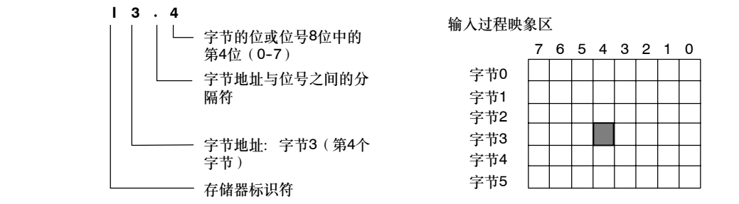
图4-3 字节.位寻址
