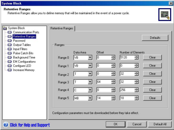
图4-21 保持存储器
