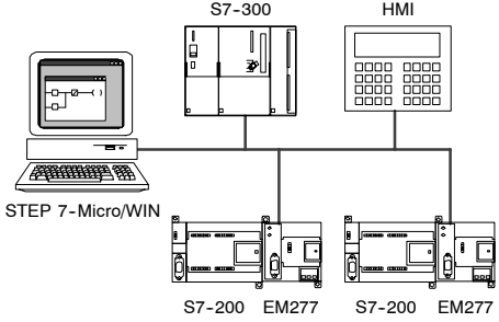
图7-16 波特率高于187.5k
