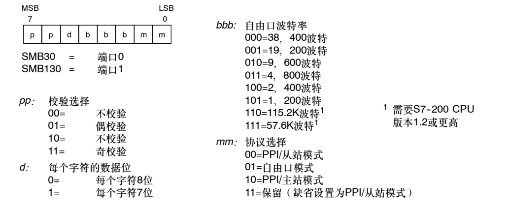
图6-8 用于自由口模式的SM控制字节（SMB30或SMB130）
