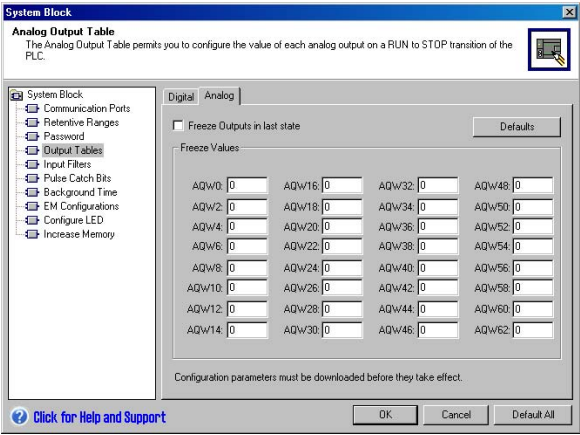
图4-20 模拟量输出表
