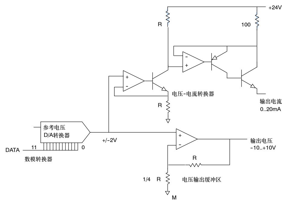
图A-18 EM232和EM235的输出方框图
