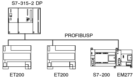
图7-17 S7-315-2 DP网络
