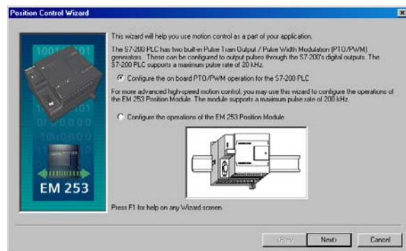
图9-2 组态PWM输出
