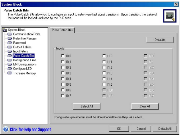
图4-24 脉冲捕捉使能
