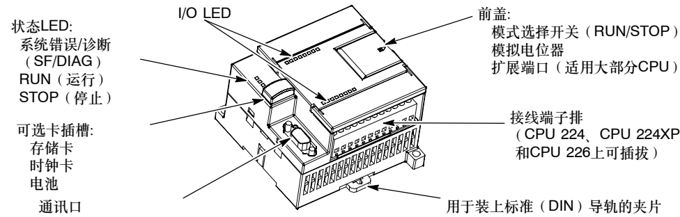
图1-1 S700微型PLC
