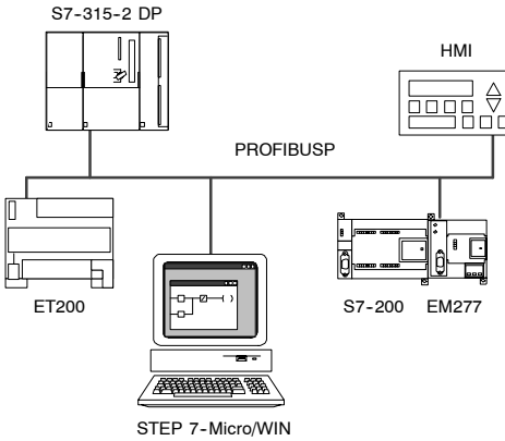
图7-18 PROFIBUS网络
