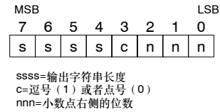
图6-20 实数转字符串指令的FMT操作数
