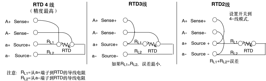
图A-22 RTD到传感器的接线，4线、3线和2线
