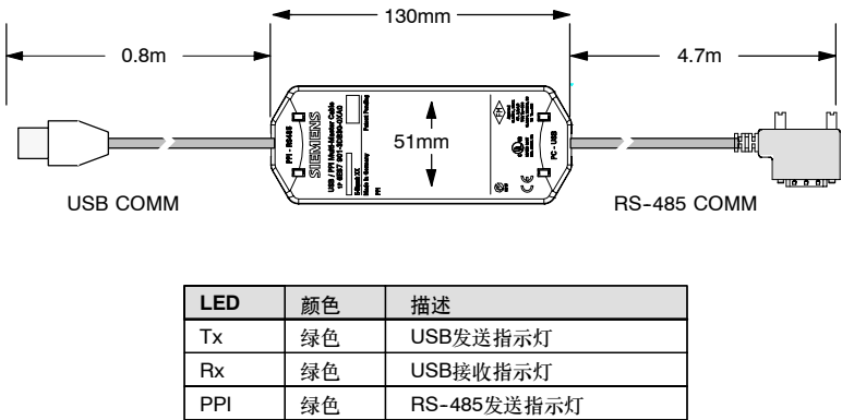
图A-42 S7-200 USB/PPI多主站电缆的尺寸和LED
