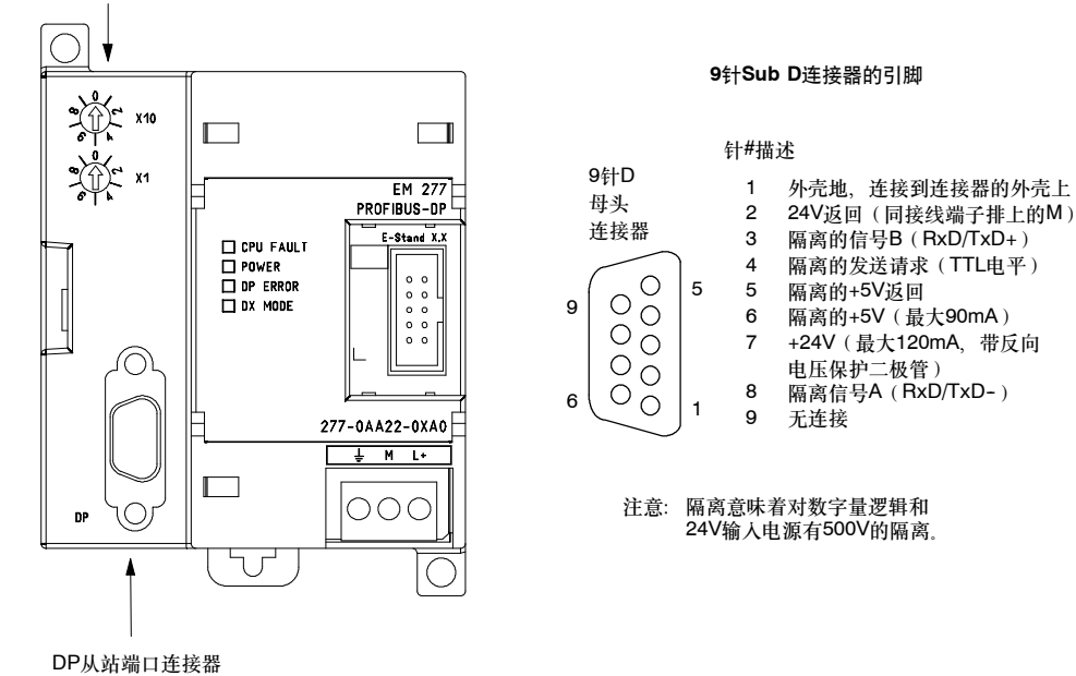
图A-23 EM277 PROFIBUS-DP
