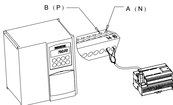
图11-6 连接到MM420的接线终端
