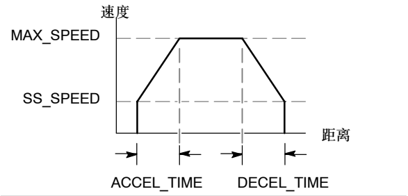
图9-5 加速和减速时间
