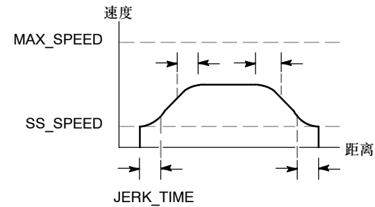
图9-14 急停补偿
