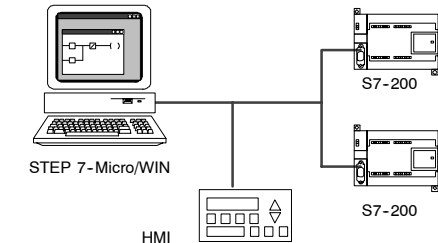
图7-12 多个主站和多个从站
