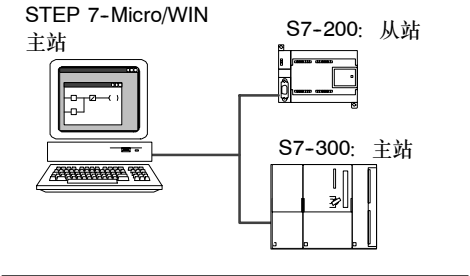
图7-8 MPI网络
