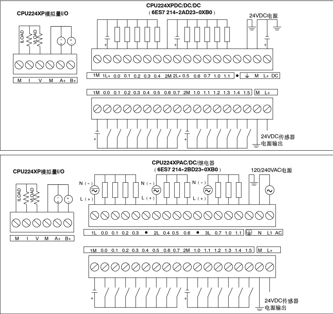
图A-5 CPU 224XP接线图
