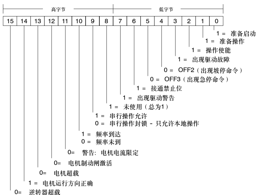
图11-4 4系列小变频标准状态字的状态位和主反馈
