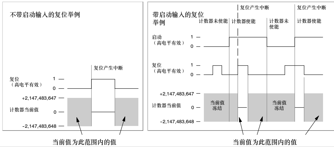
图6-27 带有或者不带启动输入的复位操作举例
