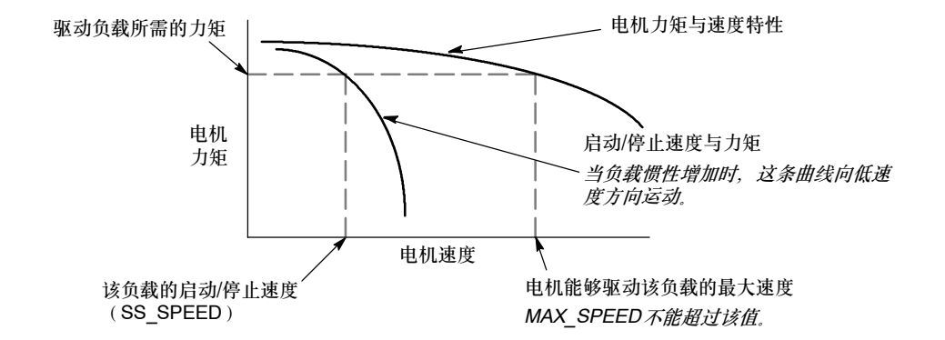
图9-4 典型电机电矩-速度曲线
