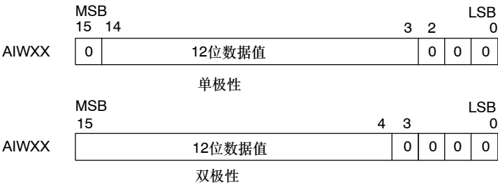
图A-14 EM231和EM235输入数据字格式
