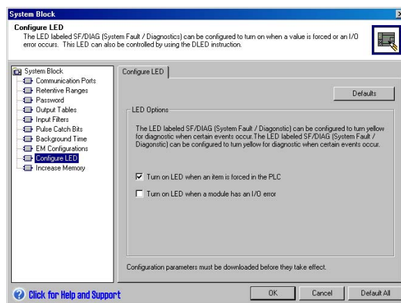
图4-28 诊断LED
