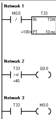
示例: STEP 7-Micro/WIN使用入门例子程序
