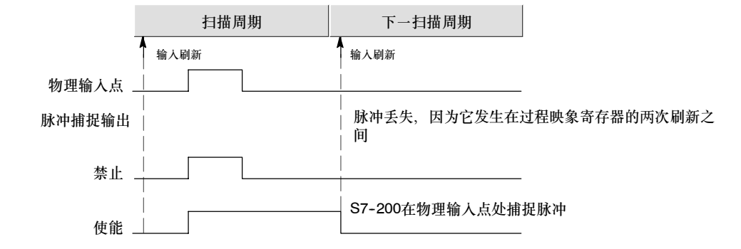
图4-25 带有和不带有脉冲捕捉功能的S7-200操作
