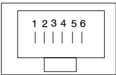
图A-30 RJ11插座的视图
