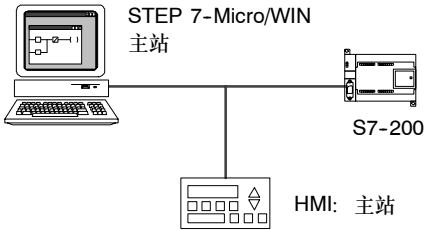
图7-7 PPI网络
