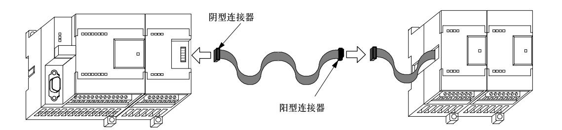
图A-40 I/O扩展电缆的典型安装
