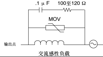
图3-4 交流负载的抑制电路
