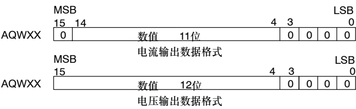
图A-17 EM231和EM235输出数据字格式
