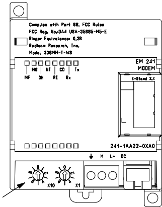
图A-29 EM241 Modem模块接线端子图
