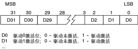
图11-2 Active参数的格式
