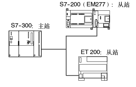
图7-9 PROFIBUS网络
