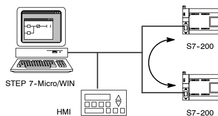
图7-13 点对点通讯
