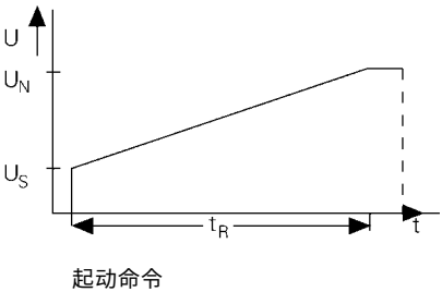
图 1 软起动电压斜坡
