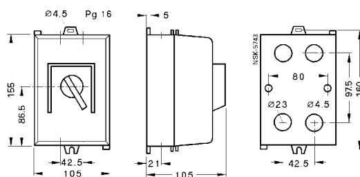
3VU9 133-2GA00 防护罩
