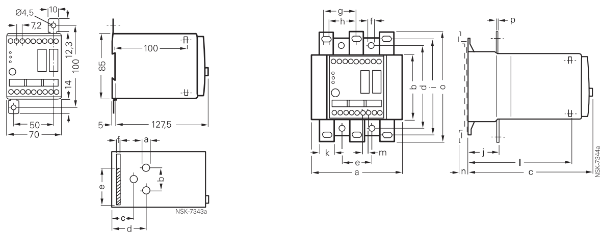
3 RB12 46 热继电器
