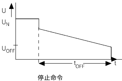
图 2 软停止电压斜坡
