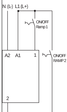
3RW31 - Dual Ramp 下图只适用于双速型 3RW1
