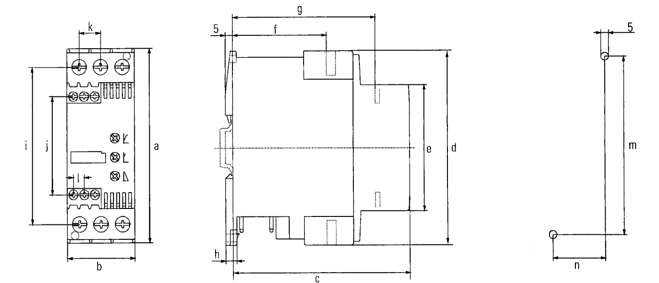
尺寸 (mm)
