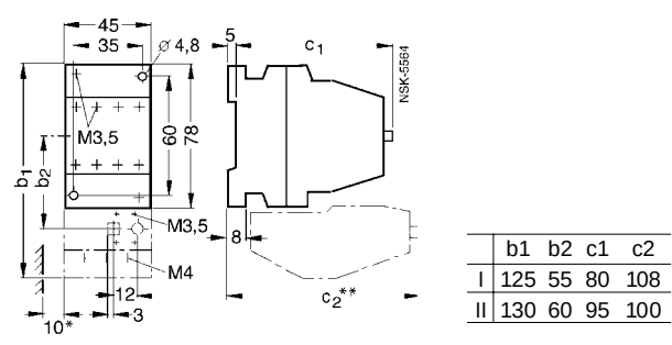
3UA50 与 3TF40/41, 3TB40/41 接触器接插安装。 (I 带有 1NO 或 1NC 辅助触头的接触器。 II 带有 1NO+1NC 或 2NO+2NC 辅助触头的接触器。)
