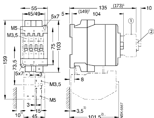
3TF34 和 3TF35, 2 级
