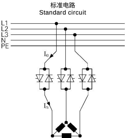
软起动器额定电流 I_e 与电动机电流 I_n 相等 3 根导体至电动机
