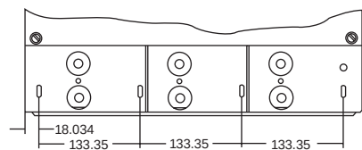
3RW3484-... 上下安装孔的位置
