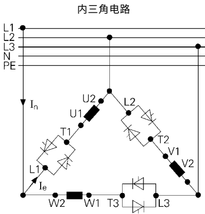
软起动器额定电流 I_e 是电动机电流 I_n 的 57% 6 根导体至电动机
