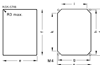
防护罩开孔尺寸
