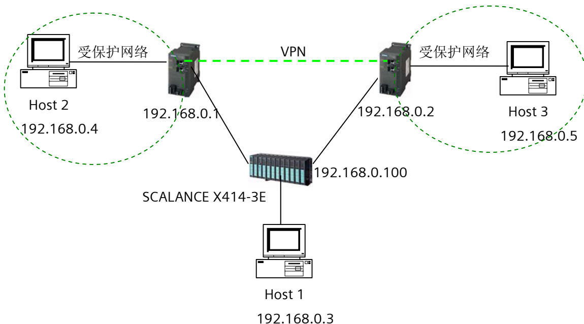
VPN 网络组态图：
