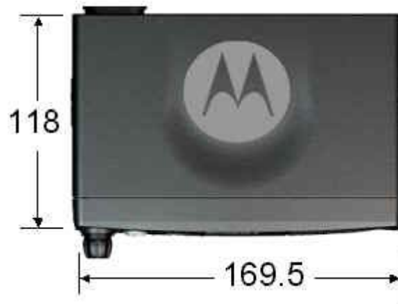
图 3 DP192G 的尺寸与接口位置图
