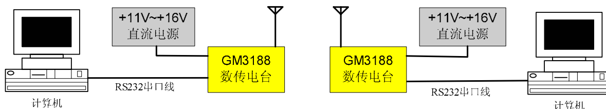
图5.GM3188-19.2K 数传电台安装示意图
