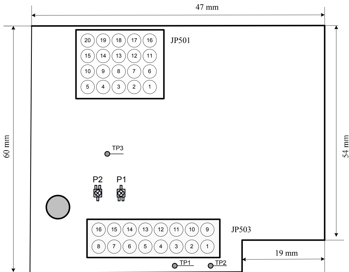
图3 DP192G 的尺寸与接口位置图
