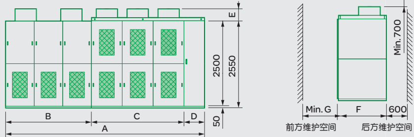
图11 10kV: 3500, 4600, 5300kVA
