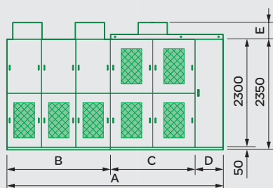
图10 10kV: 800, 1200, 1700, 2350kVA
