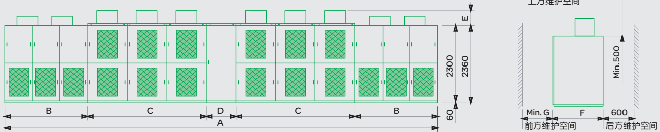
图7 6.6 kV: 7000 kVA
