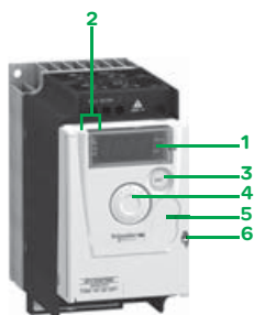
ATV12H075M2, 前面板上的门关闭, 有保护盖5: STOP/RESET(停机/复位)和RUN(运行)按钮不可用
