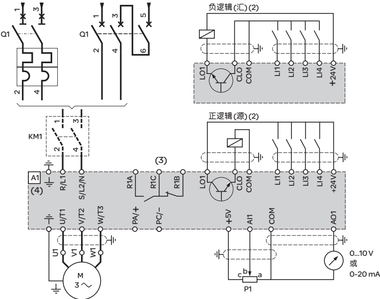
ATV 12●●●●F1, ATV 12●●●●M2 的典型接线图
