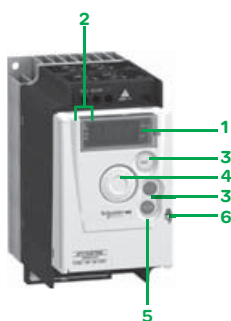
ATV12H075M2, 前面板上的门关闭, 无保护盖5: STOP/RESET(停机/复位)和RUN(运行)按钮可用
