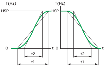
HSP：速度上限 t1 = k1 \times t2 ( k1 ：固定圆整系数) t2 ：斜坡时间设置 S 斜坡
