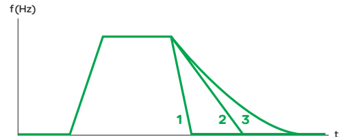
1 快速停机 2 斜坡停机 3 自由停机 停机类型
