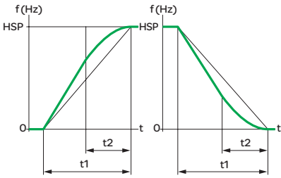
HSP：速度上限 t1 = k2 \times t2 ( k2 ：固定圆整系数) t2 ：斜坡时间设置 U 斜坡
