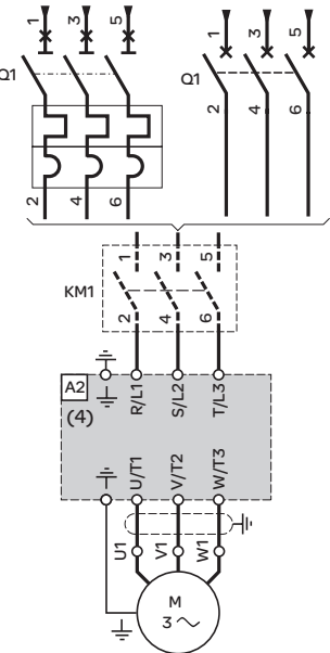
ATV 12●●●●M3 的典型接线图
