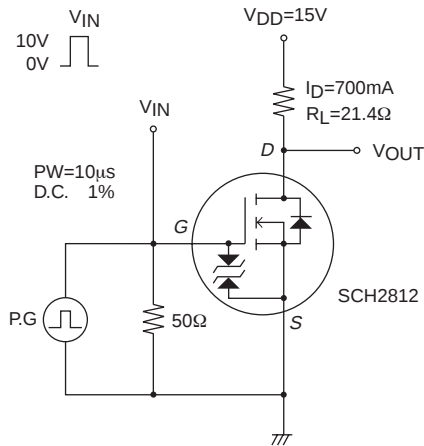
スイッチングタイム測定回路図 (MOSFET 部)
