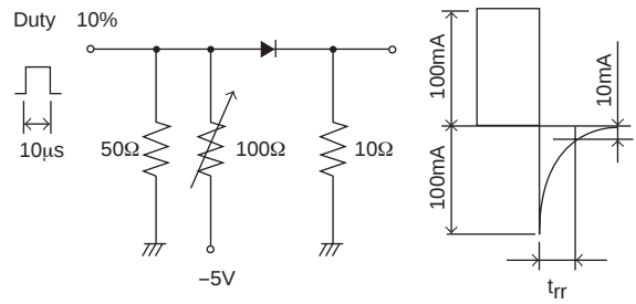
t_{rr} 指定回路図 (SBD 部)
