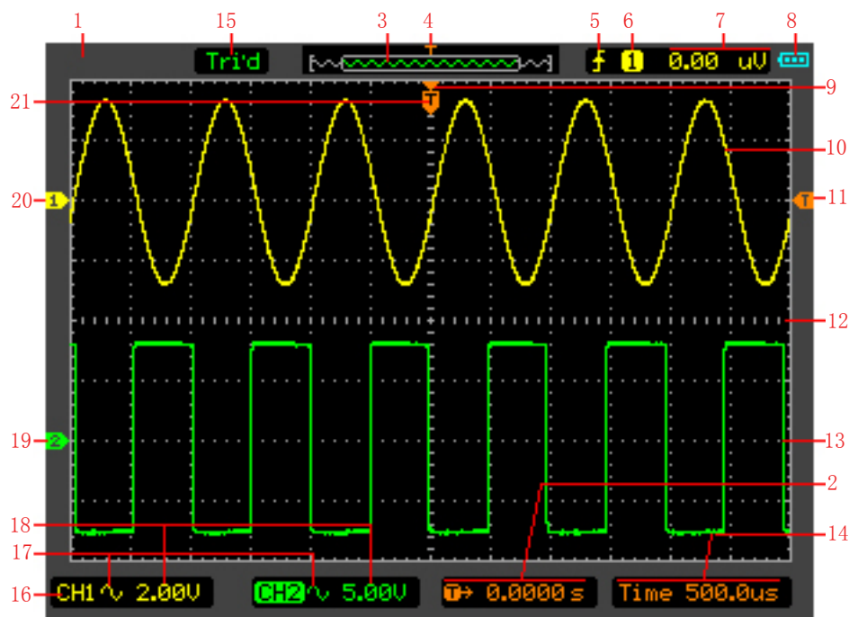
图 1-3 显示屏
