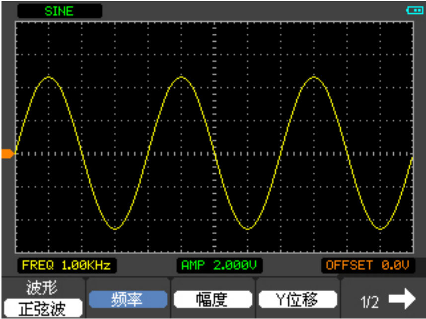
图 5-2 正弦波
