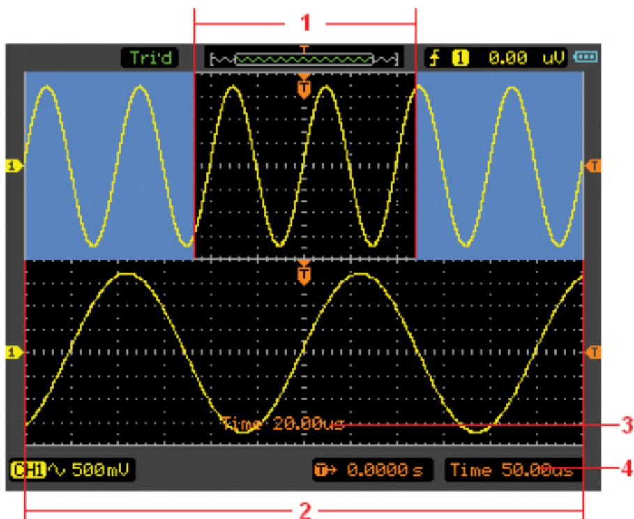
图 2-22 交替扩展
