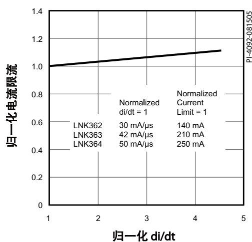
图 13. 限流点与 di/dt 的特性曲线
