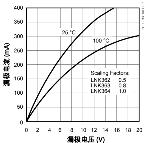
图 15. 输出特性
