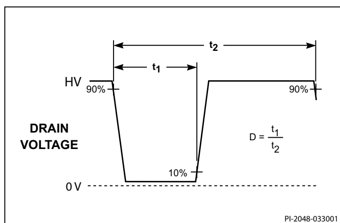
图 8. LinkSwitch-XT 占空比测量
