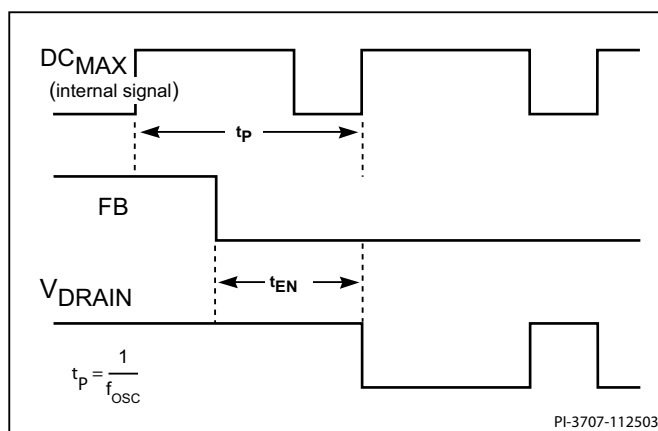
图 9. LinkSwitch-XT 输出导通定时
