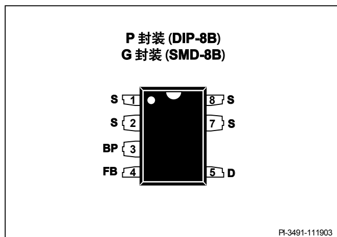
图 3. 引脚配置
