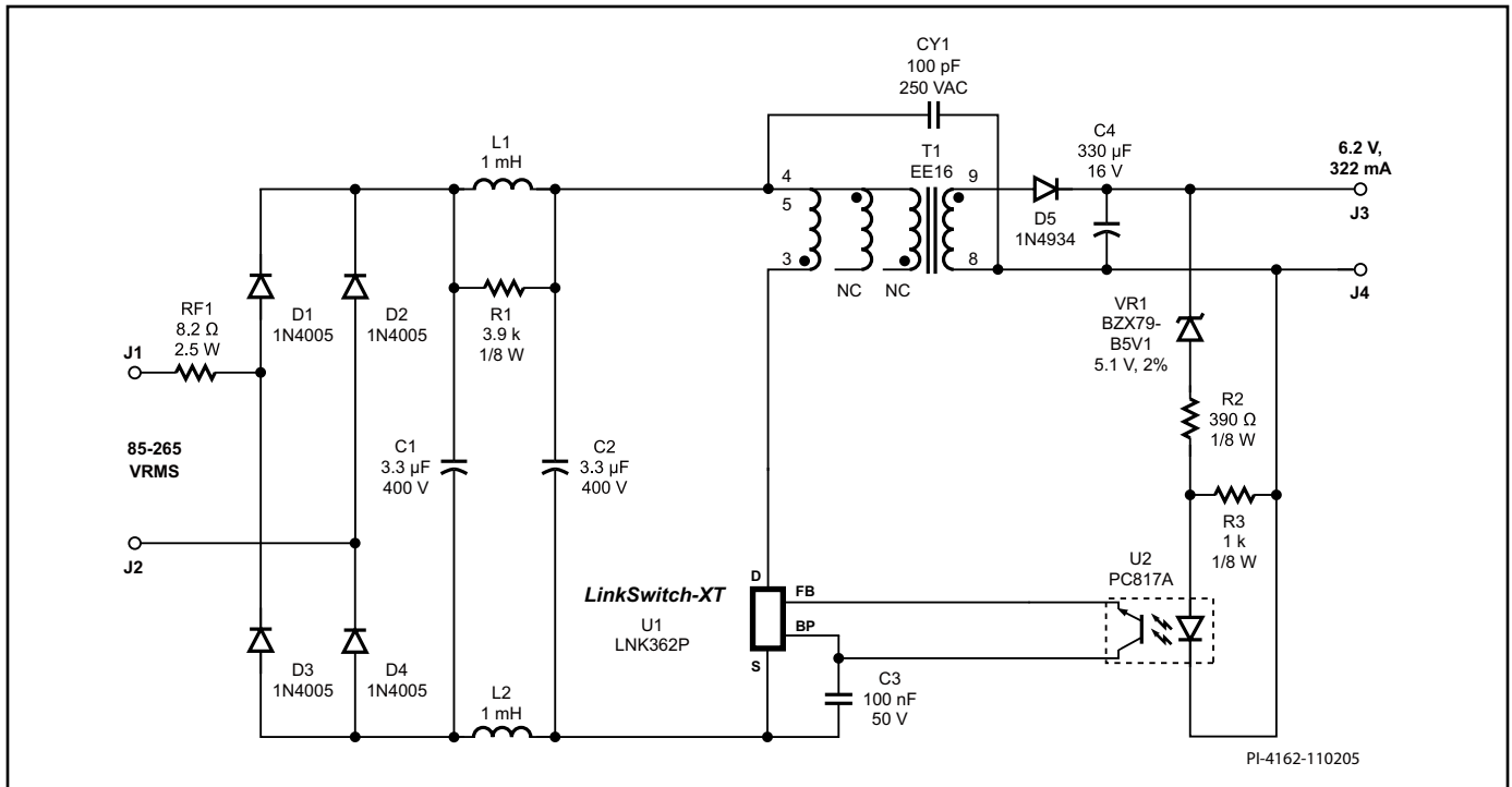
图 5. 使用LNK362的2 W通用输入电压范围CV适配器
