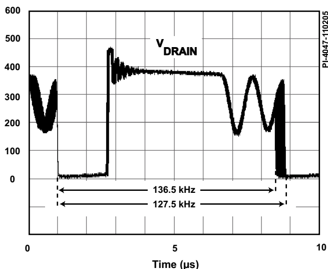
图 4. 频率抖动
