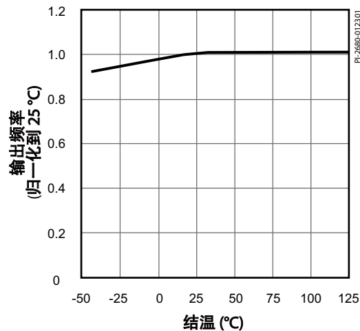
图 11. 频率与温度的特性曲线
