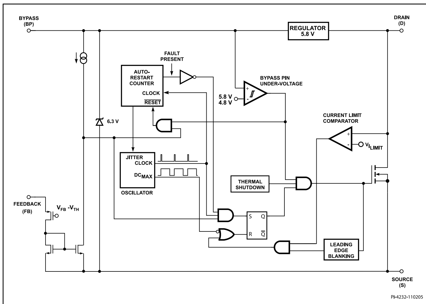
图 2. 功能结构图
