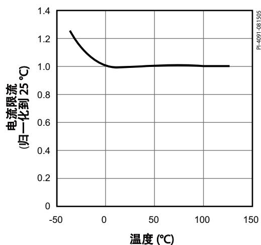
图 12. 限流点与温度的特性曲线
