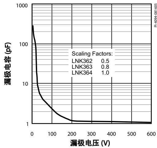
图 16. C_{OSS} 与漏极电压的曲线
