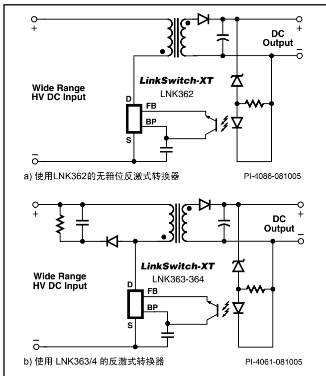
图 1. LinkSwitch-XT的典型应用
