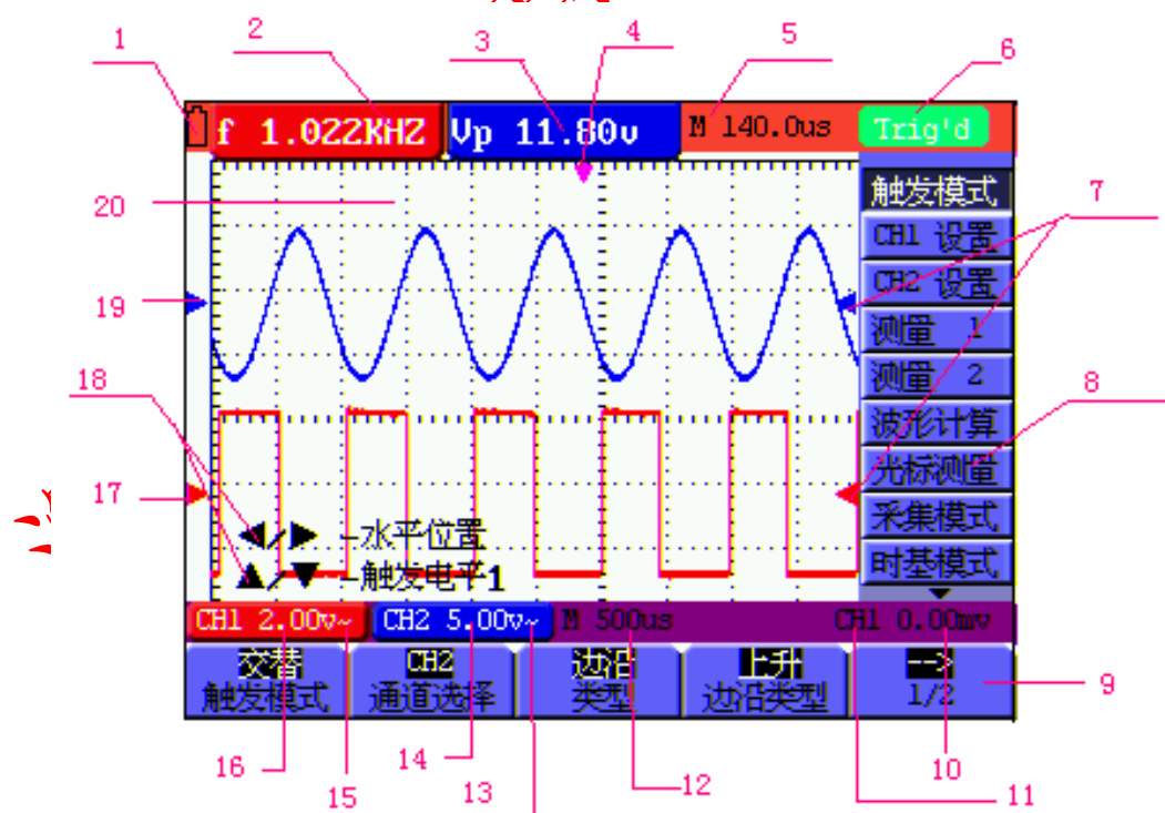
图 5: 示波器界面
