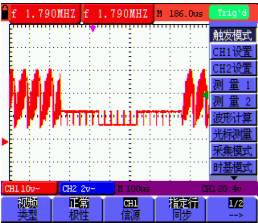
图42 视频指定行触发（第一页）
