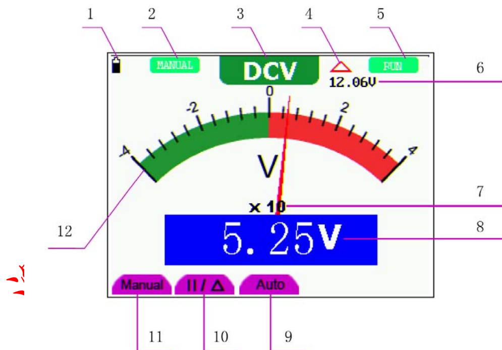
图 20：万用表界面
