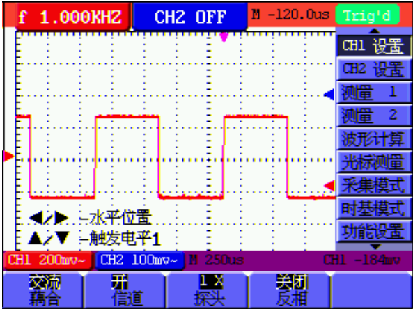
图 35：交流耦合
