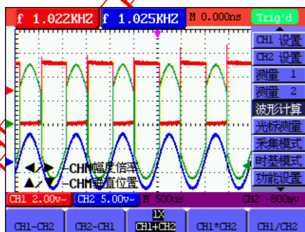
图 19: 波形计算
