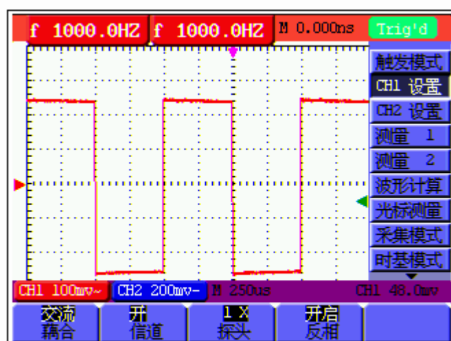
图 18: 反相开启
