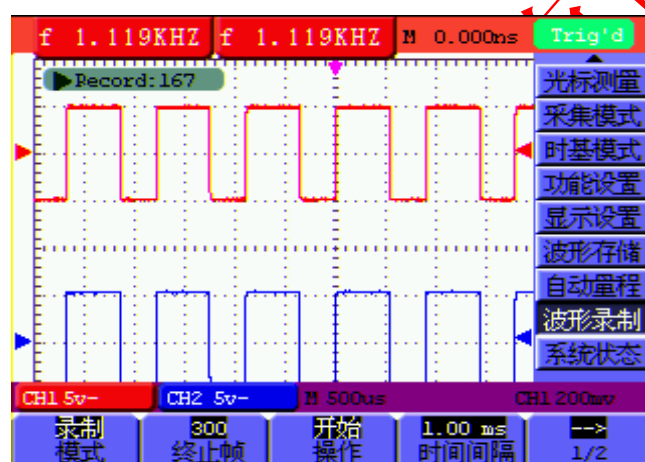
图58：波形录制第一页
