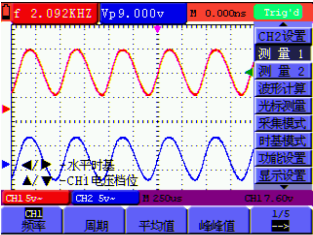
图 51：自动测量
