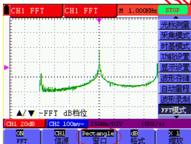
图63. RECTANGLE 窗
