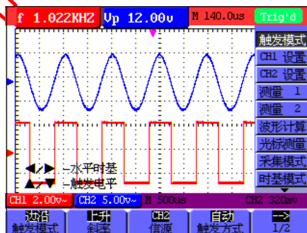
图 39：边沿触发
